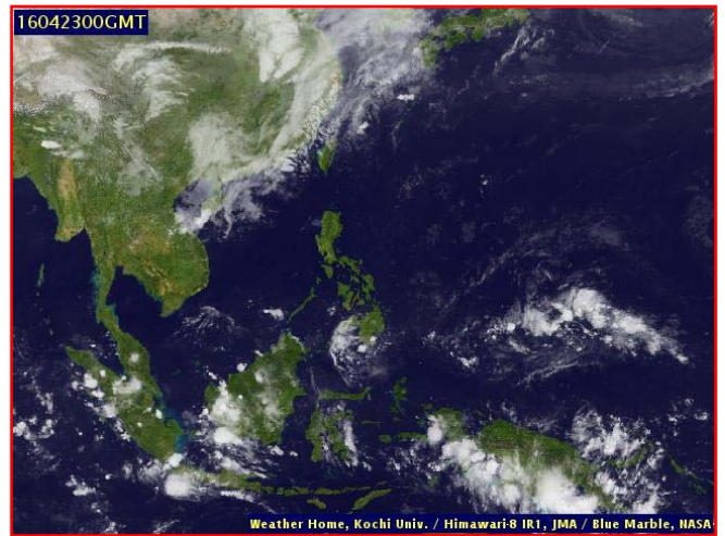
ภาพถ่ายจากดาวเทียม วันที่ ๒๓ เม.ย. ๒๕๕๙ เวลา ๐๗.๐๐ น.
