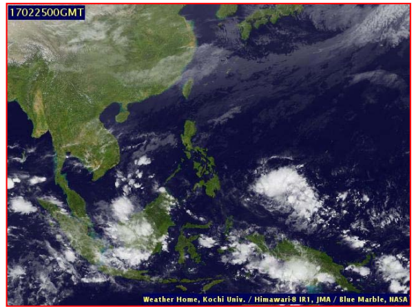
ภาพถ่ายจากดาวเทียม วันที่ ๒๕ ก.พ. ๒๕๖๐ เวลา ๐๗.๐๐ น.
