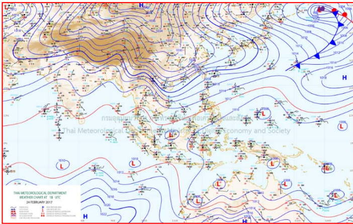
แผนที่อากาศ วันที่ ๒๕ ก.พ. ๒๕๖๐ เวลา ๐๖.๐๐ น.
