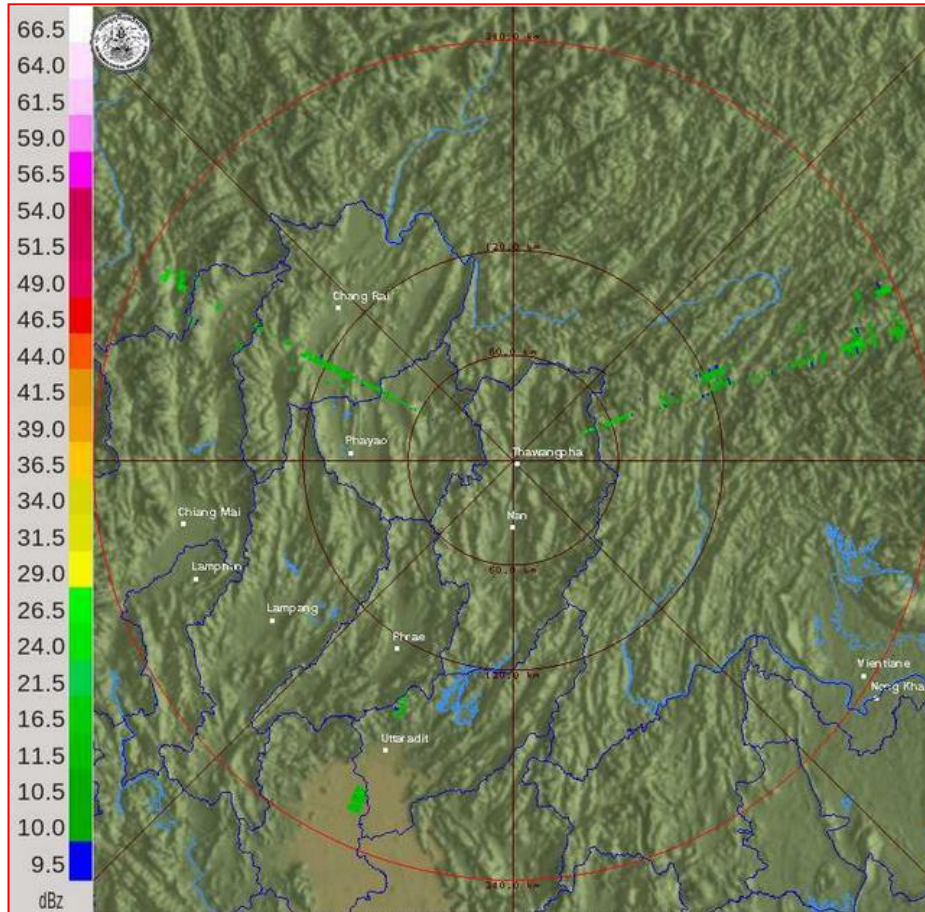
ภาพเรดาร์ตรวจอากาศ “น่าน” ณ วันที่ 22 กุมภาพันธ์ 2560 (ที่มา : กรมอุตุนิยมวิทยา)
