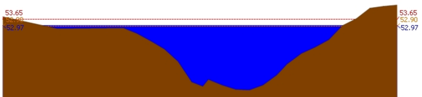
สถานี 120113T แม่น้ำป่าสักที่บ้านเขาค้าง อ.คลองกระเจิง อ.ศรีเทพ จ.เพชรบูรณ์ ระดับน้ำ 52.97 ม.รทก.
