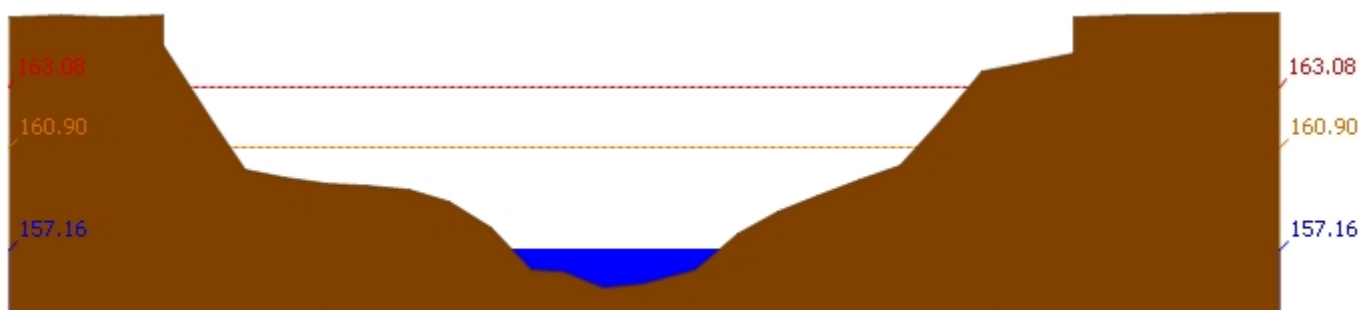
สถานี 120105T แม่น้ำป่าสักที่บ้านวังมลิเหิน อ.ท่าอิฐ จ.พิษณุโลก ระดับน้ำ 157.16 ม.รทก.
