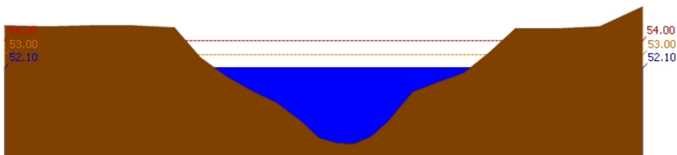
สถานี 120702T ลำสนธิที่บ้านท่าช้าง ต.หนองขาหย่าง อ.ชัยบาดาล จ.ลพบุรี ระดับน้ำ 52.10 ม.รทก.
