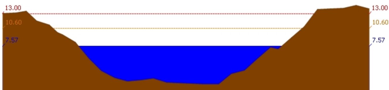
สถานี 120106T แม่น้ำป่าสักที่ อ.เสาไห้ ต.ศาลาวิไทย อ.เสาไห้ จ.สระบุรี ระดับน้ำ 7.57 ม.รทก.
