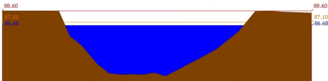
สถานี 120110T แม่น้ำป่าสักที่บ้านวังโบสถ์ ต.วังโบสถ์ อ.หนองไผ่ จ.เพชรบูรณ์ ระดับน้ำ 86.68 ม.รทก.
