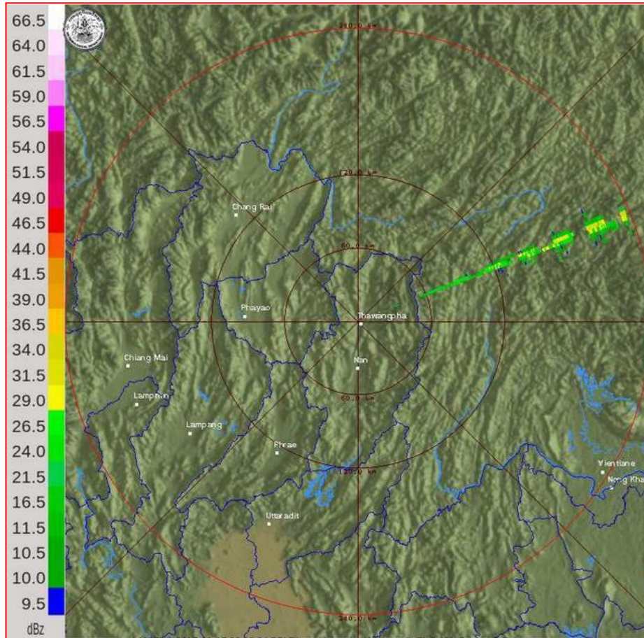
ภาพเรดาร์ตรวจอากาศ “น่าน” ณ วันที่ 17 มกราคม 2560 (ที่มา : กรมอุตุนิยมวิทยา)
