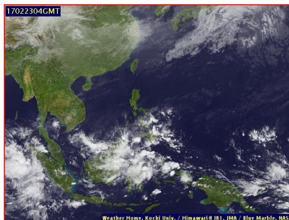
ภาพถ่ายจากดาวเทียม วันที่ 23 ก.พ. 2560
