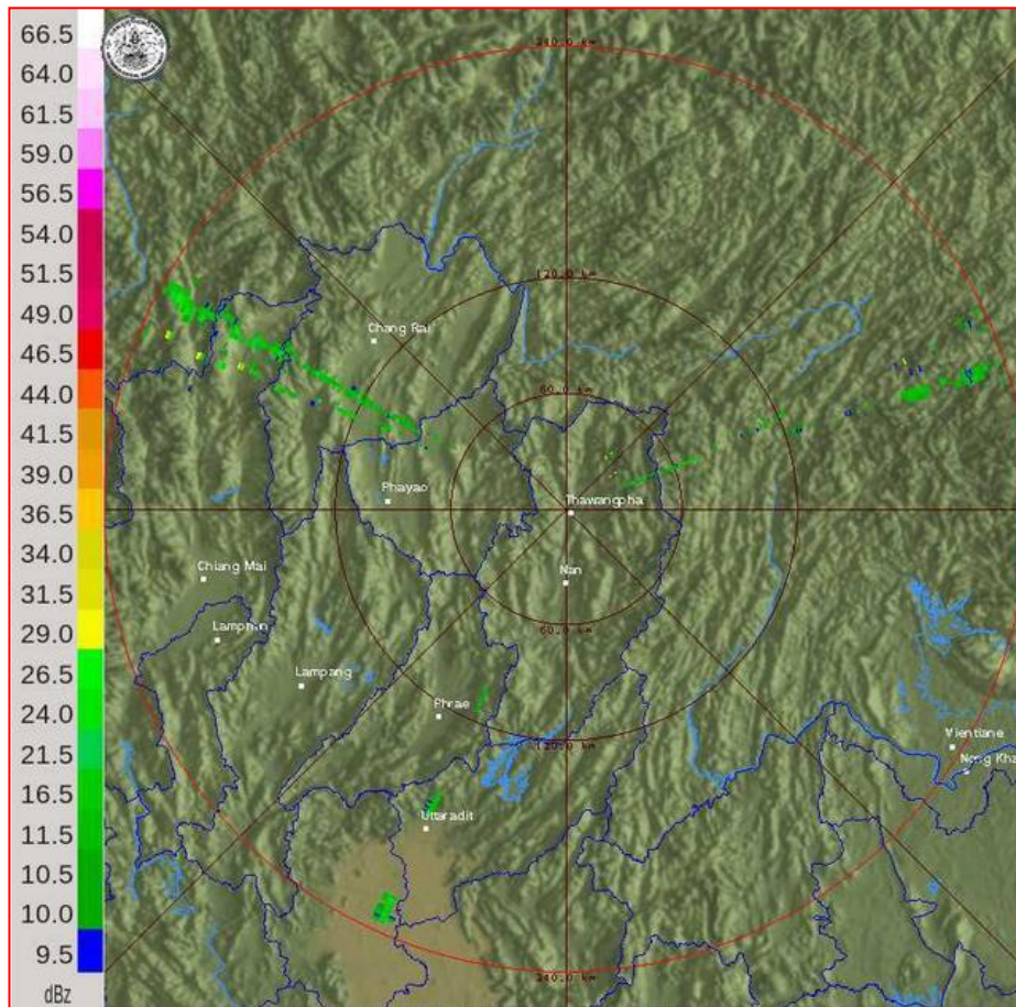
ภาพเรดาร์ตรวจอากาศ “น่าน” ณ วันที่ 23 กุมภาพันธ์ 2560 (ที่มา : กรมอุตุนิยมวิทยา)
