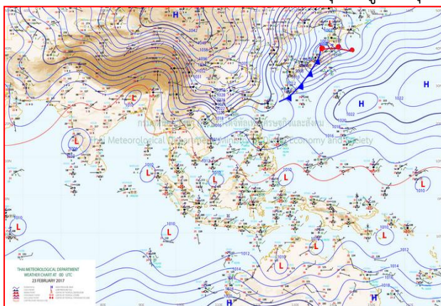
แผนที่อากาศ วันที่ 23 ก.พ. 2560 เวลา 07.00 น.
