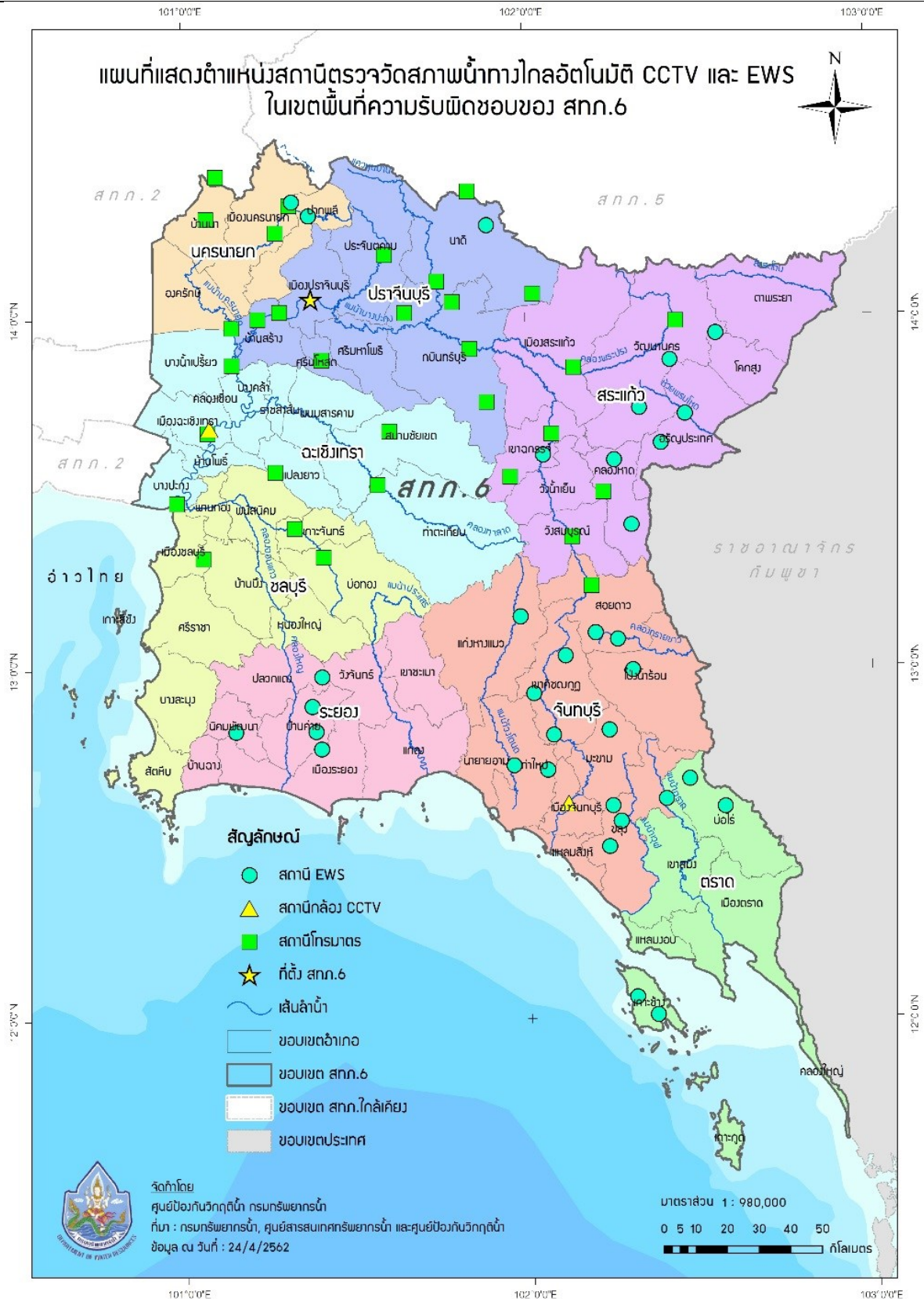
รูปที่ 4 ตำแหน่งสถานีตรวจวัดสภาพน้ำทางไกลอัตโนมัติ CCTV และ EWS ในเขตพื้นที่ความรับผิดชอบของสำนักงานทรัพยากรน้ำภาค 6
