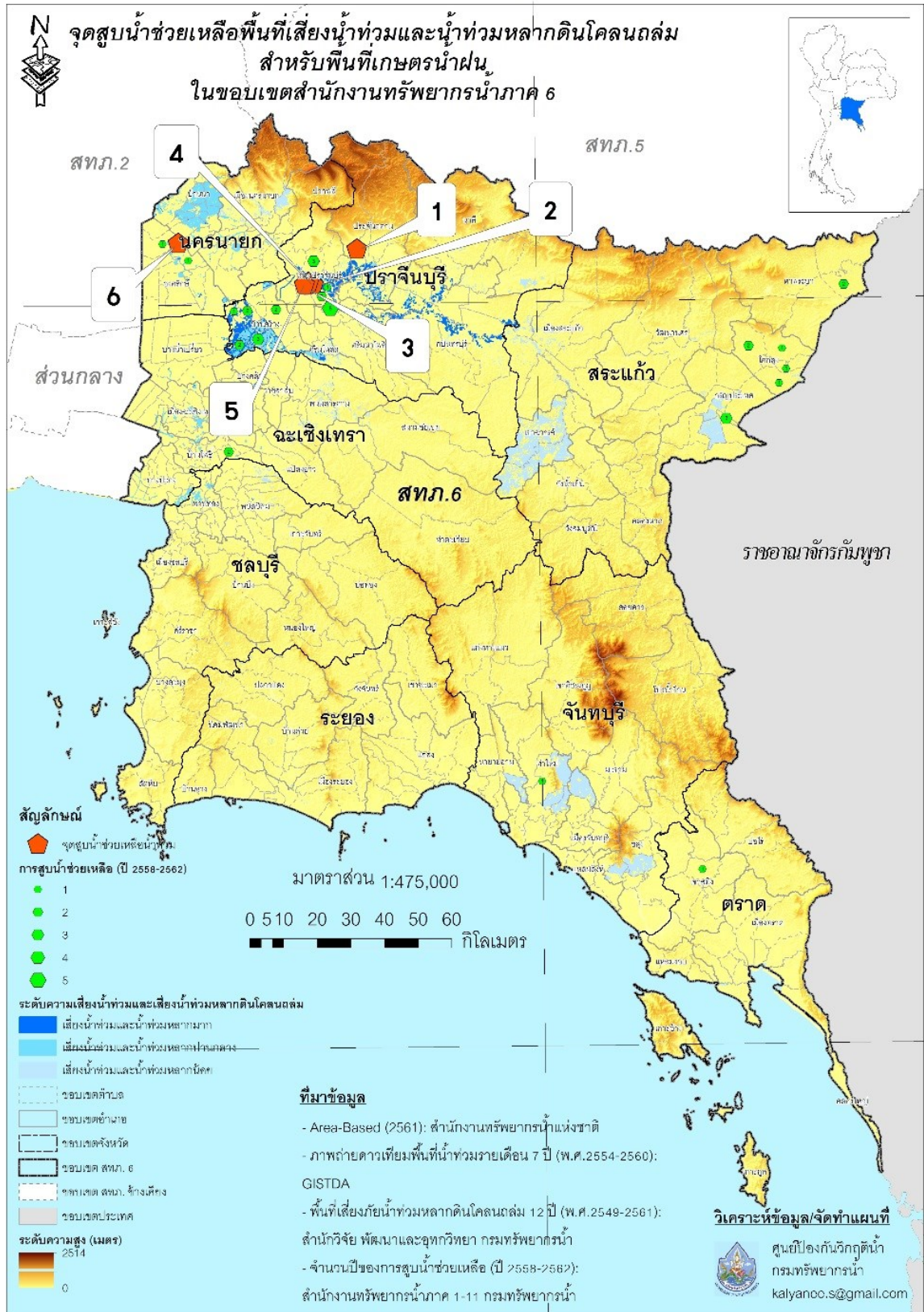
รูปที่ 6 ตำแหน่งจุดติดตั้งเครื่องสูบน้ำ ช่วยเหลือน้ำท่วมช่วงเดือนมิถุนายน – ธันวาคม ในเขตพื้นที่ที่ความรับผิดชอบของสำนักงานทรัพยากรน้ำภาค 6
