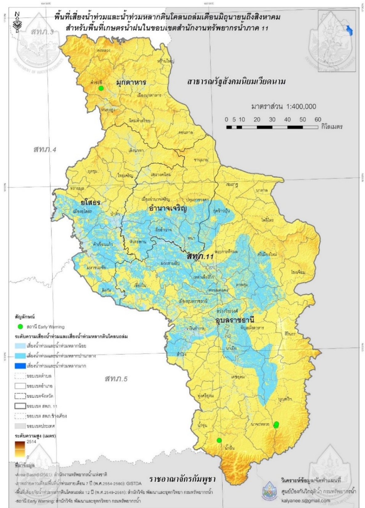
รูปที่ 2 พื้นที่เสี่ยงน้ำท่วมและน้ำท่วมหลากดินถล่มระหว่างเดือนมิถุนายนถึงสิงหาคม สำหรับพื้นที่เขตนํ้าฝนในขอบเขตสำนักงานทรัพยากรน้ำภาค 11
