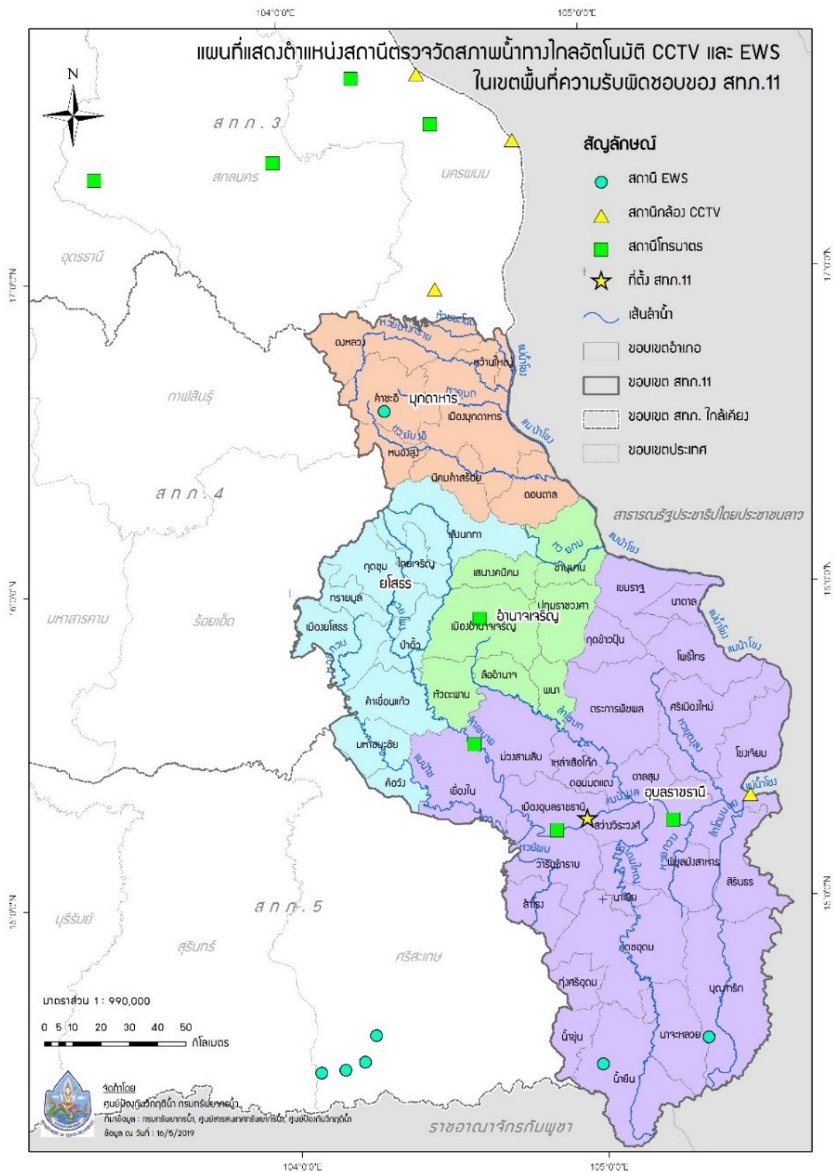
รูปที่ 5 ตำแหน่งสถานีตรวจวัดสภาพน้ำทางไกลอัตโนมัติ CCTV และ EWS ในเขตพื้นที่ความรับผิดชอบของสำนักงานทรัพยากรน้ำภาค 11
