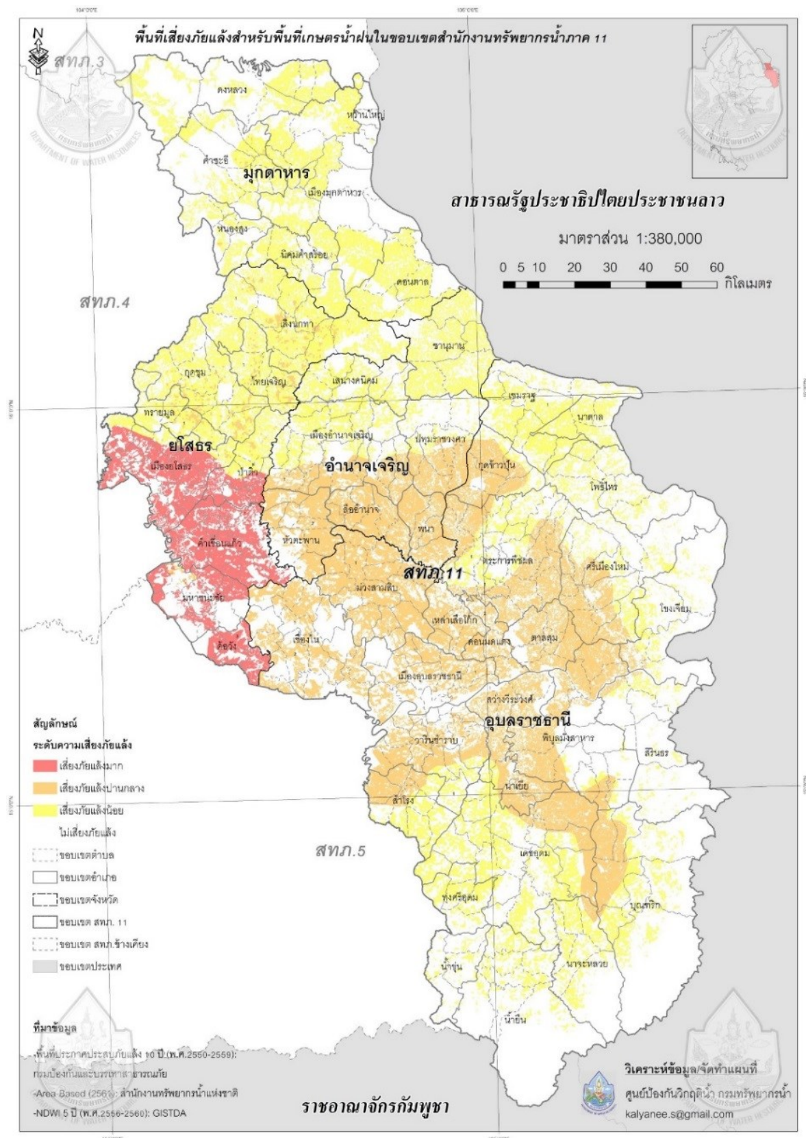
รูปที่ 4 พื้นที่เสี่ยงภัยแล้งสำหรับพื้นที่เกษตรน้ำฝนในขอบเขตสำนักงานทรัพยากรน้ำภาค 11
