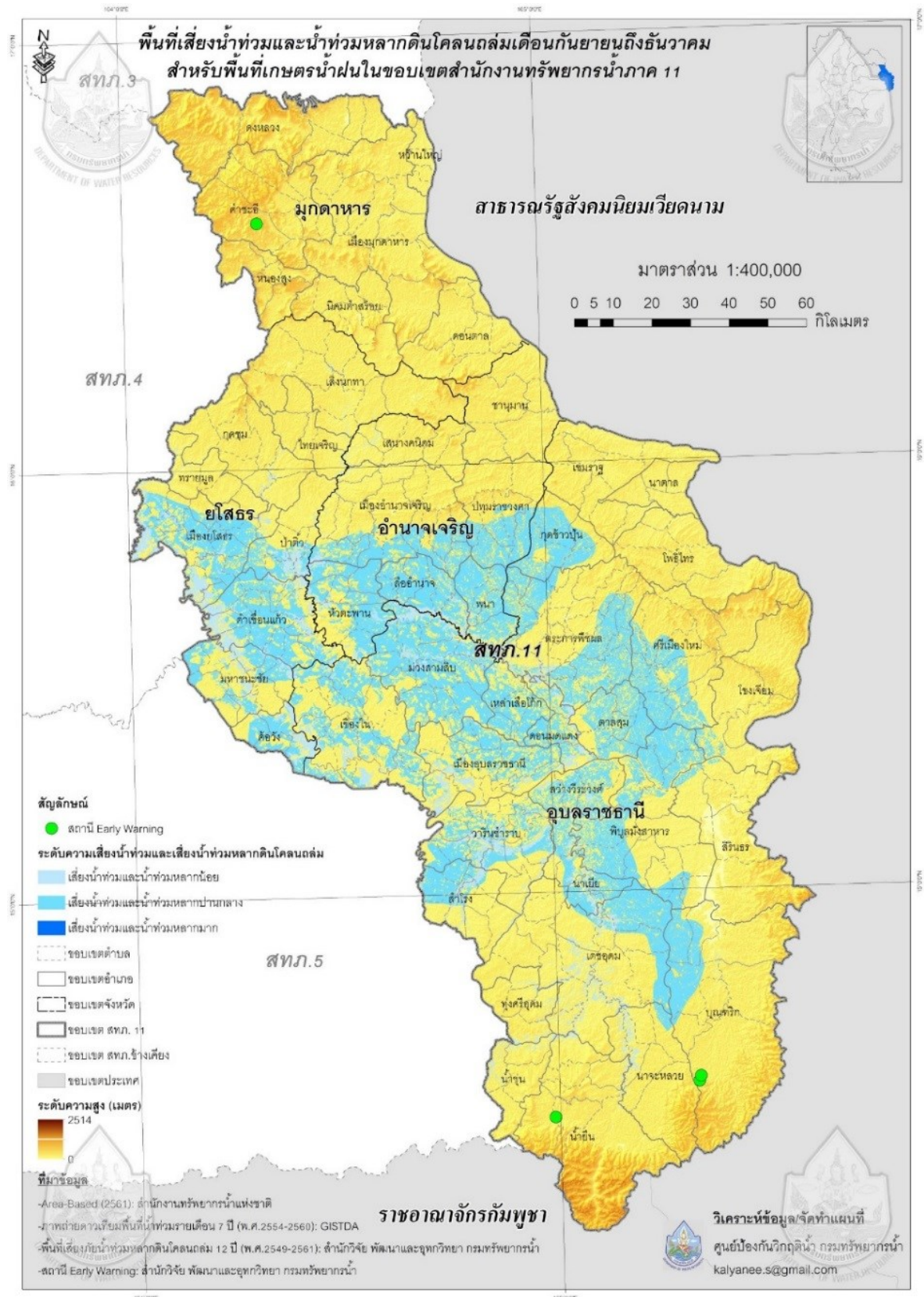
รูปที่ 3 พื้นที่เสี่ยงน้ำท่วมและน้ำท่วมหลากดินโคลนถล่มระหว่างเดือนกันยายนถึงธันวาคม สำหรับพื้นที่เกษตรน้ำฝนในขอบเขตสำนักงานทรัพยากรน้ำภาค 11
