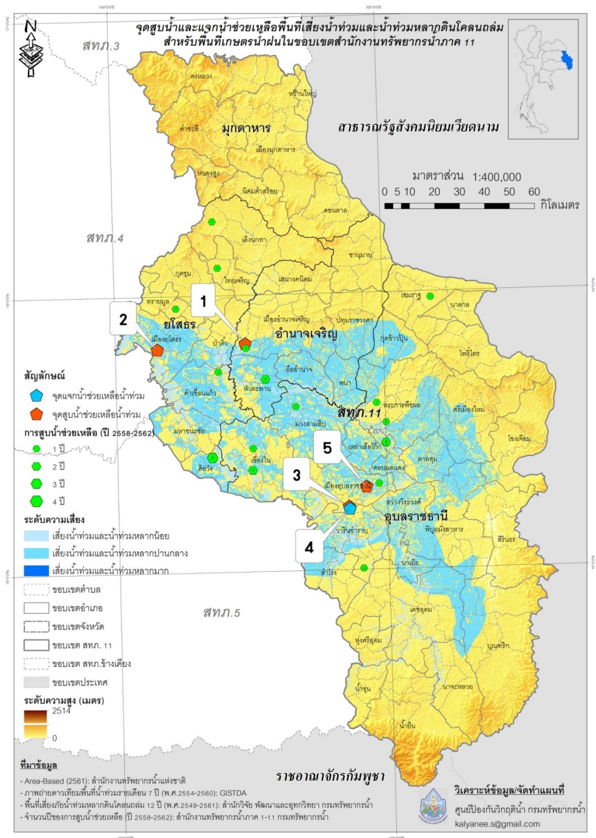
รูปที่ 7 ตำแหน่งจุดติดตั้งเครื่องสูบน้ำ ช่วยเหลือน้ำท่วมช่วงเดือนมิถุนายน – ธันวาคม ในเขตพื้นที่ความรับผิดชอบของสำนักงานทรัพยากรน้ำภาค 11
