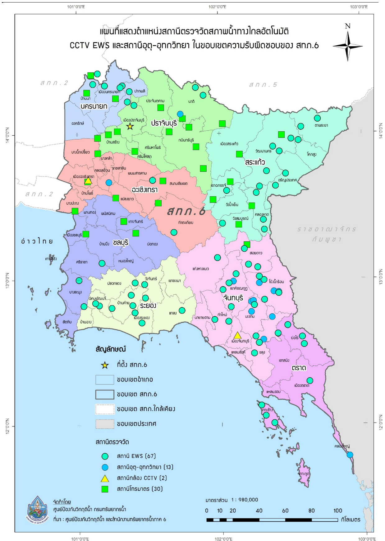
รูปที่ 3 ตำแหน่งสถานีตรวจวัดสภาพน้ำทางไกลอัตโนมัติ CCTV EWS และสถานีอุตุ-อุทกวิทยา ในเขตพื้นที่ความรับผิดชอบของสำนักงานทรัพยากรน้ำภาค 6
