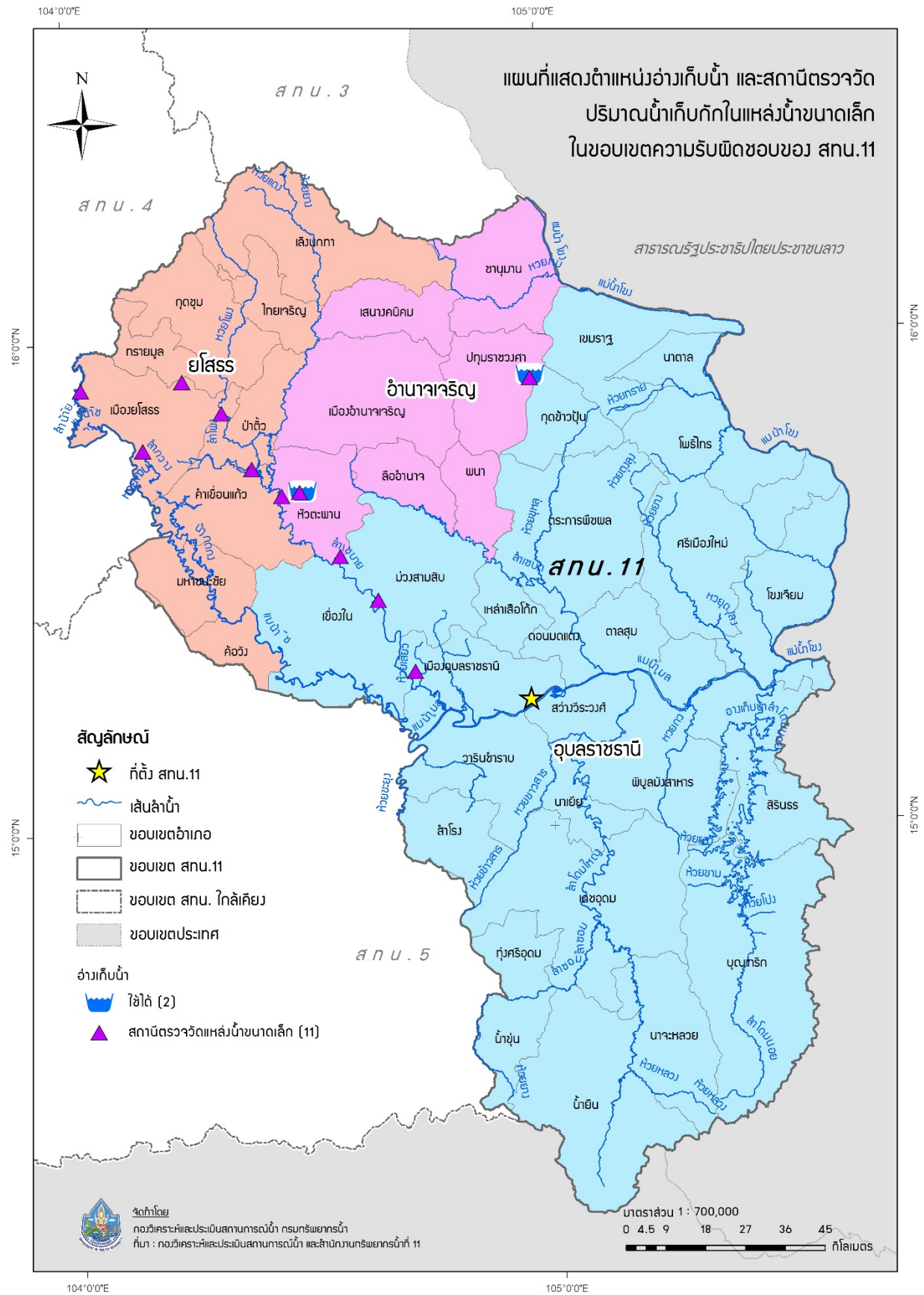
รูปที่ 4 ตำแหน่งโครงการพัฒนาแหล่งน้ำประเภทอ่างเก็บน้ำในเขตพื้นที่ความรับผิดชอบของ สำนักงานทรัพยากรน้ำที่ 11
