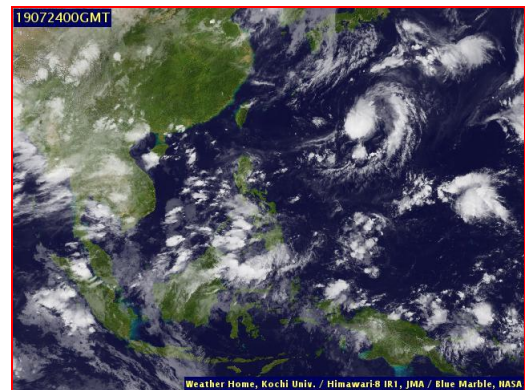
ภาพถ่ายจากดาวเทียม วันที่ 24 ก.ค. 2562
