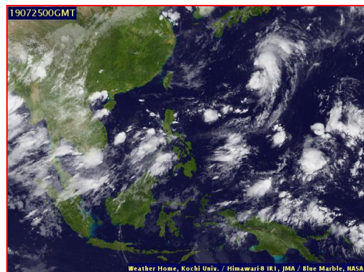
ภาพถ่ายจากดาวเทียม วันที่ 25 ก.ค. 2562
