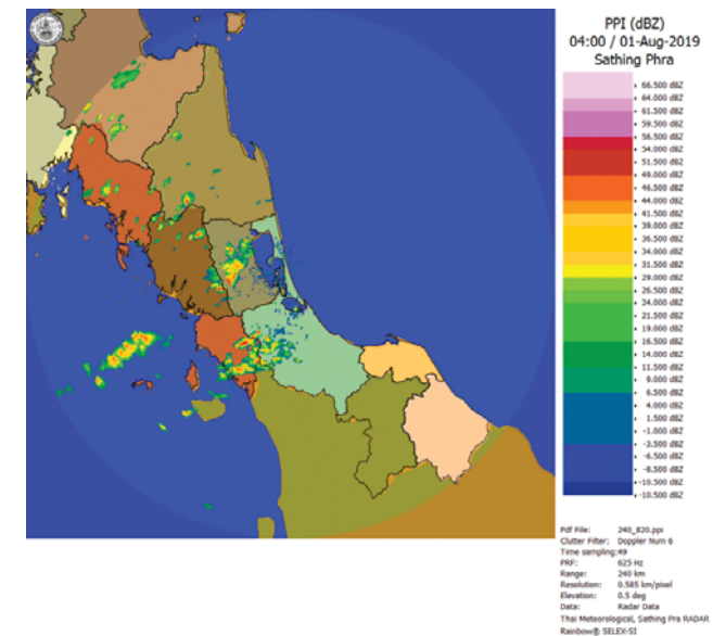
ภาพเรดาร์ตรวจอากาศ "สทิงพระ" ณ วันที่ 1 สิงหาคม 2562 (ที่มา : กรมอุตุนิยมวิทยา)
