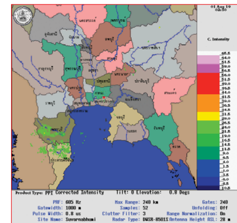
ภาพเรดาร์ตรวจอากาศ “สถานีสุวรรณภูมิ” ณ วันที่ 1 สิงหาคม 2562 เวลา 09.30 น. (ที่มา : กรมอุตุนิยมวิทยา)
