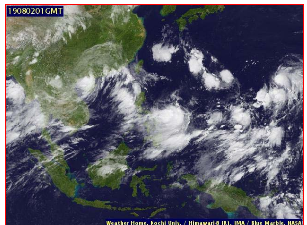
ภาพถ่ายดาวเทียม วันที่ ๒ ส.ค. ๒๕๖๒ เวลา ๐๘.๐๐ น.
