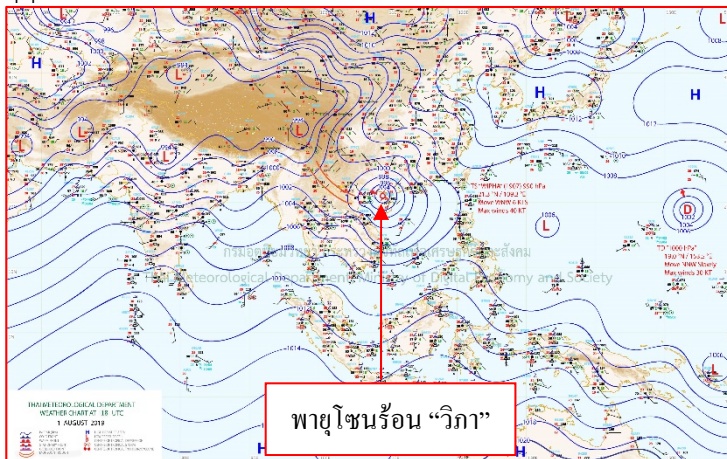
แผนที่อากาศ วันที่ ๒ ส.ค. ๒๕๖๒ เวลา ๐๑.๐๐ น.
