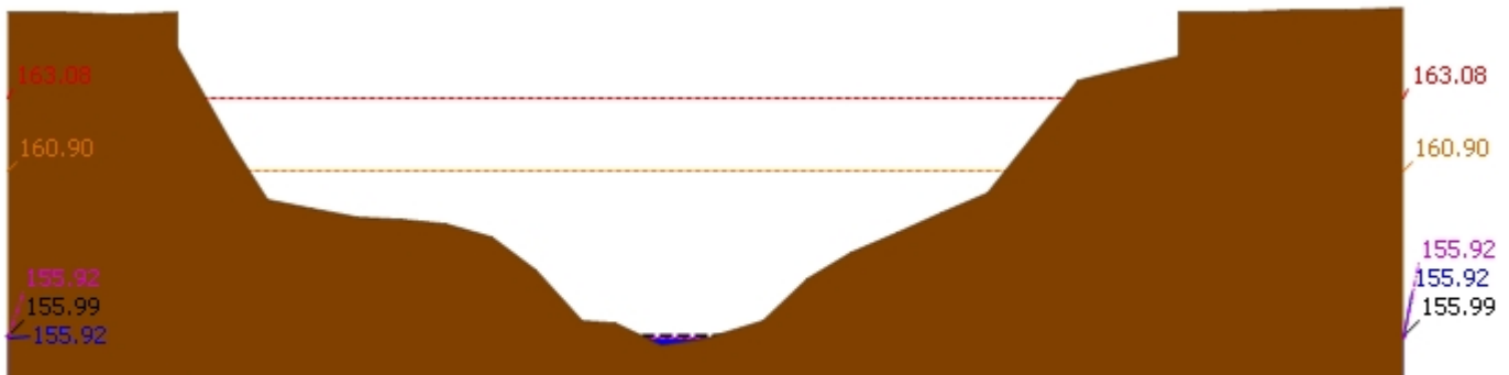
▲ ระดับปัจจุบัน --- ระดับวิกฤติ --- ระดับเฟิาระวัง ---- เมื่อวาน 7:00 น. - - - - - คาดการณ์ล่วงหน้า 1 วัน สถานี 120105T แม่น้ำป่าสักที่บ้านวังมเสหนือ ต.ทำอัญญ อ.หล่มสัก จ.เพชรบูรณ์ ระดับน้ำ 155.92 ม.รทก.
