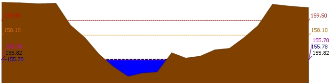
▲ ระดับปัจจุบัน --- ระดับวิกฤติ --- ระดับเฟิาระวัง ---- เมื่อวาน 7:00 น. - - - - - คาดการณ์ล่วงหน้า 1 วัน สถานี 120305T หัวน้ำพุ่งที่ อ.หล่มเก่า ต.หล่มเก่า อ.หล่มเก่า จ.เพชรบูรณ์ ระดับน้ำ 155.78 ม.รทก.
