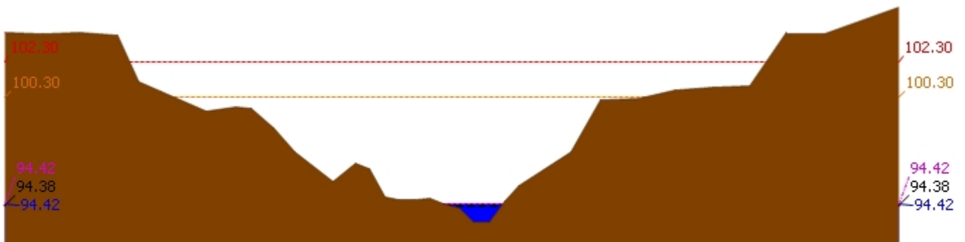
▲ ระดับปัจจุบัน --- ระดับวิกฤติ --- ระดับเฟิาระวัง ---- เมื่อวาน 7:00 น. - - - - - คาดการณ์ล่วงหน้า 1 วัน สถานี 120112T แม่น้ำป่าสักที่บ้านหนองแหวน ต.วังมะข่อ อ.เมือง จ.เพชรบูรณ์ ระดับน้ำ 94.42 ม.รทก.
