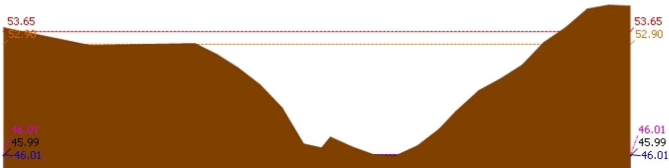
▲ ระดับปัจจุบัน --- ระดับวิกฤติ --- ระดับเฝ้าระวัง ---- เมื่อวาน 7:00 น. - - - - - คาดการณ์ล่วงหน้า 1 วัน สถานี 120113T แม่น้ำป่าสักที่บ้านเขาค้าง ต.คลองกระจิง อ.ศรีเทพ จ.เพชรบูรณ์ ระดับน้ำ 46.01 ม.รทก.
