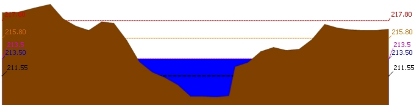
▲ ระดับปัจจุบัน --- ระดับวิกฤติ --- ระดับเฟิาระวัง ---- เมื่อวาน 7:00 น. - - - - คาคตการลลวงหน้า 1 วัน สถานี 120205T แม่น้ำป่าสักที่ บ้านอุ่มกะทาด ต.ศิลา อ.หล่มเก่า จ.เพชรบูรณ์ ระดับน้ำ 213.50 ม.รทก.
