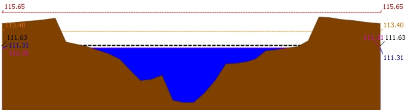
▲ ระดับปัจจุบัน --- ระดับวิกฤติ --- ระดับเฟิาระวัง ---- เมื่อวาน 7:00 น. - - - - คาคตการลลวงหน้า 1 วัน สถานี 120107T แม่น้ำป่าสักที่ อ.เมืองเพชรบูรณ์ ต.นาป่า อ.เมือง จ.เพชรบูรณ์ ระดับน้ำ 111.31 ม.รทก.
