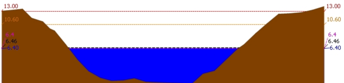
▲ ระดับปัจจุบัน --- ระดับวิกฤติ --- ระดับฝายระวัง ---- เมื่อกวาน 7:00 น. - - - - คาดการณ์ล่วงหน้า 1 วัน สถานี 120106T แม่น้ำป่าสักที่ อ.เสาไห้ ต.ศาลารีไทย อ.เสาไห้ จ.สระบุรี ระดับน้ำ 6.40 ม.รทก.
