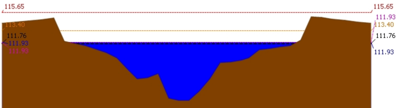
▲ ระดับปัจจุบัน --- ระดับวิกฤติ --- ระดับฝายระวัง ---- เมื่อกวาน 7:00 น. - - - - คาดการณ์ล่วงหน้า 1 วัน สถานี 120107T แม่น้ำป่าสักที่ อ.เมืองเพชรบูรณ์ ต.นาป่า อ.เมือง จ.เพชรบูรณ์ ระดับน้ำ 111.93 ม.รทก.
