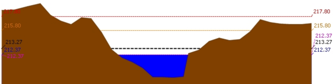
▲ ระดับปัจจุบัน --- ระดับวิกฤติ --- ระดับฝายระวัง ---- เมื่อกวาน 7:00 น. - - - - คาดการณ์ล่วงหน้า 1 วัน สถานี 120205T แม่น้ำป่าสักที่บ้านอุมกะทาด ต.ศิลา อ.หล่มเก่า จ.เพชรบูรณ์ ระดับน้ำ 212.37 ม.รทก.
