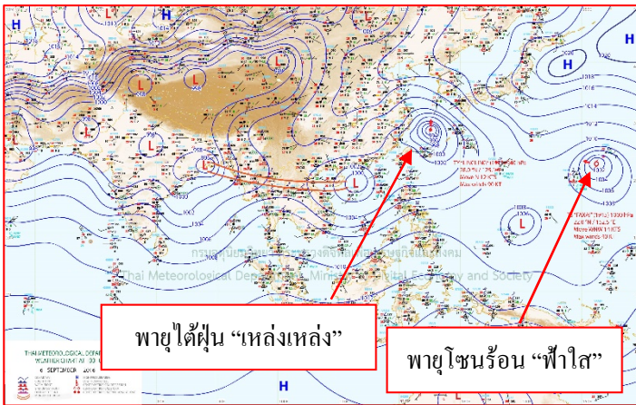
แผนที่อากาศ วันที่ ๖ ก.ย. ๒๕๖๒ เวลา ๐๗.๐๐ น.
