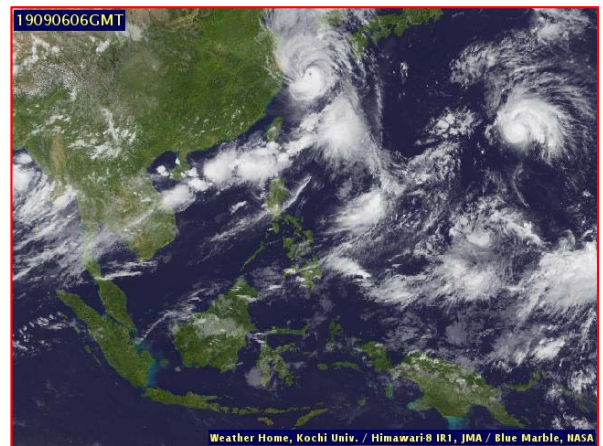
ภาพถ่ายดาวเทียม วันที่ ๖ ก.ย. ๒๕๖๒ เวลา ๑๓.๐๐ น.
