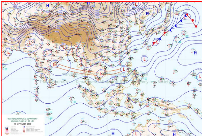
แผนที่อากาศ วันที่ ๑๗ ก.ย. ๒๕๖๒ เวลา ๐๗.๐๐ น.
