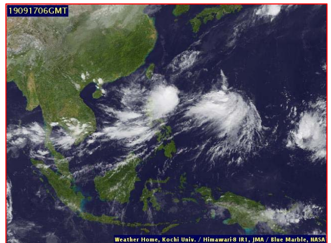
ภาพถ่ายดาวเทียม วันที่ ๑๗ ก.ย. ๒๕๖๒ เวลา ๑๓.๐๐ น.
