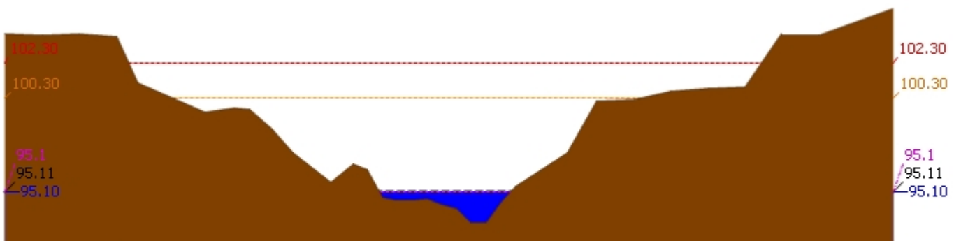
▲ ระดับปัจจุบัน --- ระดับวิกฤติ --- ระดับฝายระวัง ---- เมื่อวาน 7:00 น. - - - - - คาดการณ์ล่วงหน้า 1 วัน สถานี 120112T แม่น้ำป่าสักที่บ้านหนองแหวน ต.วังมะข่อ อ.เมือง จ.เพชรบูรณ์ ระดับน้ำ 95.10 ม.รทก.
