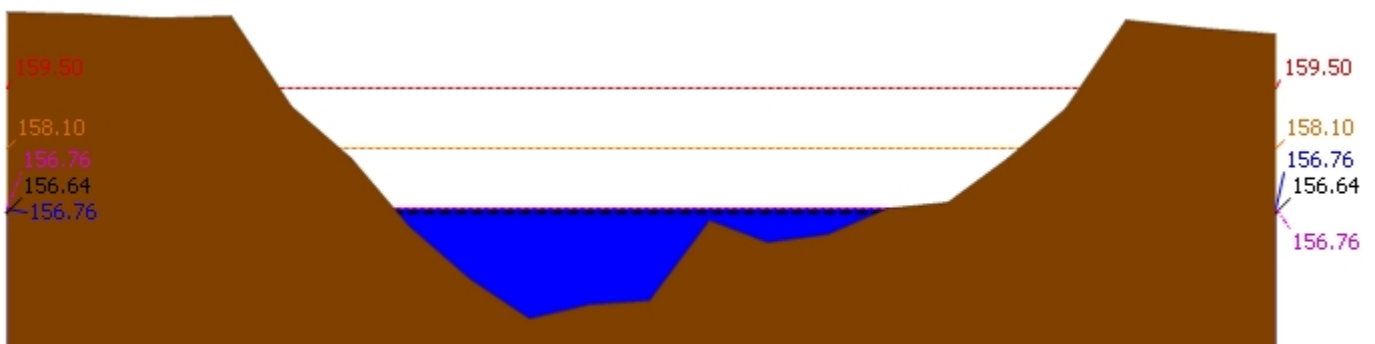
▲ ระดับปัจจุบัน --- ระดับวิกฤติ --- ระดับฝายระวัง ---- เมื่อวาน 7:00 น. - - - - - คาดการณ์ล่วงหน้า 1 วัน สถานี 120305T หัวน้ำพุอยู่ที่ อ.หล่มเก่า ต.หล่มเก่า อ.หล่มเก่า จ.เพชรบูรณ์ ระดับน้ำ 156.76 ม.รทก.
