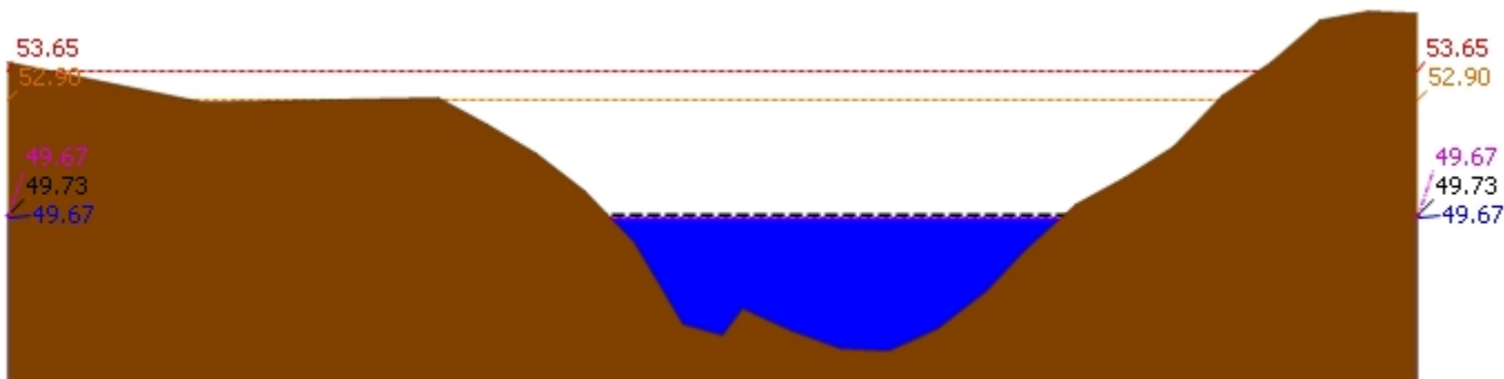
▲ ระดับปัจจุบัน --- ระดับวิกฤติ --- ระดับเฝ้าระวัง ---- เมื่อวาน 7:00 น. - - - - คาดการณ์ล่วงหน้า 1 วัน สถานี 120113T แม่น้ำป่าสักที่บ้านเขาค้าง ต.คลองกระจิง อ.ศรีเทพ จ.เพชรบูรณ์ ระดับน้ำ 49.67 ม.รทก.
