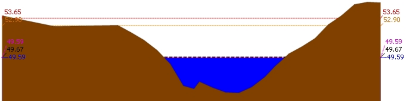
▲ ระดับปัจจุบัน --- ระดับวิกฤติ --- ระดับเฝ้าระวัง ---- เมื่อกวาน 7:00 น. - - - - คาดการณ์ล่วงหน้า 1 วัน สถานี 120113T แม่น้ำป่าสักที่บ้านเขาค้าง ต.คลองกระจิง อ.ศรีเทพ จ.เพชรบูรณ์ ระดับน้ำ 49.59 ม.รทก.
