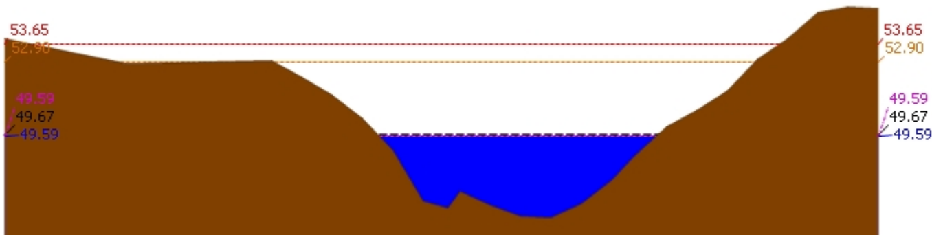
▲ ระดับปัจจุบัน --- ระดับวิกฤติ --- ระดับฝายระวัง ---- เมื่อวาน 7:00 น. - - - - - คาดการณ์ล่วงหน้า 1 วัน สถานี 120113T แม่น้ำป่าสักที่บ้านเขาค้าง ต.คลองกระจิง อ.ศรีเทพ จ.เพชรบูรณ์ ระดับน้ำ 49.59 ม.รทก.
