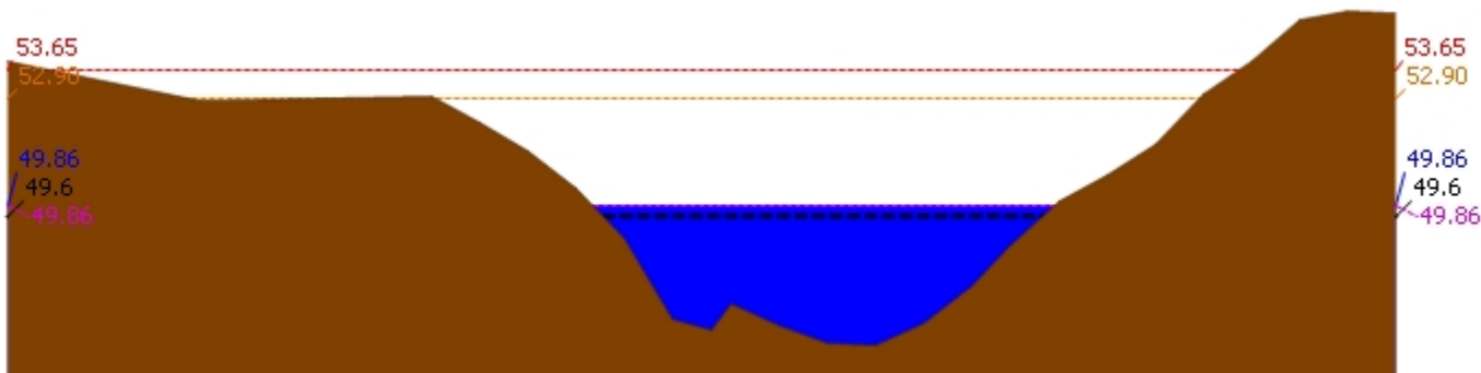
▲ ระดับปัจจุบัน --- ระดับวิกฤติ --- ระดับเฝ้าระวัง ---- เมื่อวาน 7:00 น. - - - - คาดการณ์ล่วงหน้า 1 วัน สถานี 120113T แม่น้ำป่าสักที่บ้านเขาค้าง ต.คลองกระจิง อ.ศรีเทพ จ.เพชรบูรณ์ ระดับน้ำ 49.86 ม.รทก.
