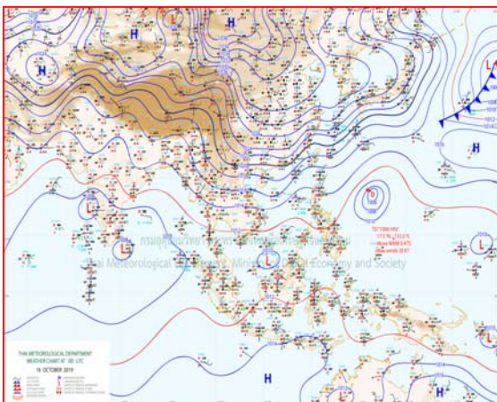
แผนที่อากาศ วันที่ 16 ต.ค. 2562 เวลา 07.00 น.
