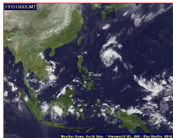
ภาพถ่ายจากดาวเทียม วันที่ 16 ต.ค. 2562
