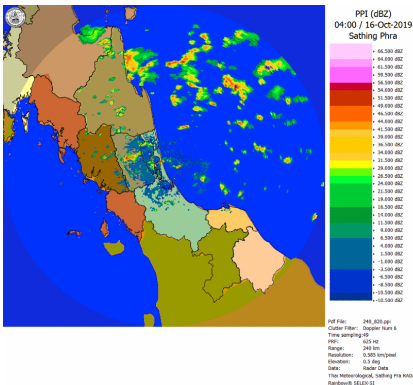
ภาพเรดาร์ตรวจอากาศ “สทิงพระ” ณ วันที่ 16 ตุลาคม 2562 (ที่มา : กรมอุตุนิยมวิทยา)
