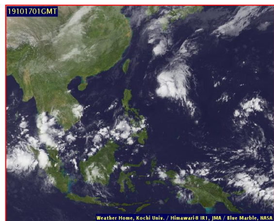
ภาพถ่ายจากดาวเทียม วันที่ 17 ต.ค. 2562
