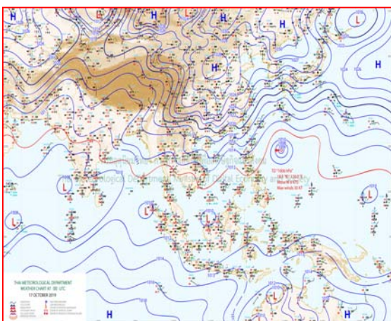
แผนที่อากาศ วันที่ 17 ต.ค. 2562 เวลา 07.00 น.
