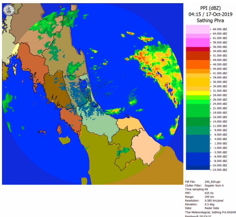
ภาพเรดาร์ตรวจอากาศ “สทิงพระ” ณ วันที่ 17 ตุลาคม 2562 (ที่มา : กรมอุตุนิยมวิทยา)
