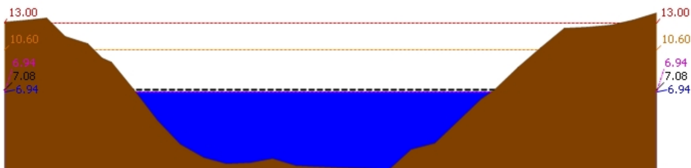
▲ ระดับปัจจุบัน --- ระดับวิกฤติ --- ระดับเฟิาระวัง ---- เมื่อกาน 7:00 น. - - - - - คาดการณ์ล่วงหน้า 1 วัน สถานี 120106T แม่น้ำป่าสักที่ อ.เสาไห้ ต.ศาลารีย์ไทย อ.เสาไห้ จ.สระบุรี ระดับน้ำ 6.94 ม.รทก.
