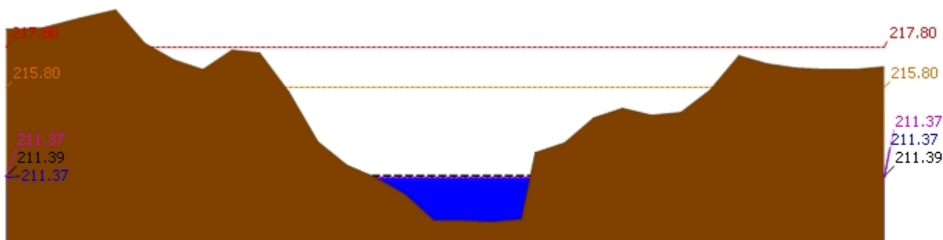
▲ ระดับปัจจุบัน --- ระดับวิกฤติ --- ระดับเฟิาระวัง ---- เมื่อกาน 7:00 น. - - - - - คาดการณ์ล่วงหน้า 1 วัน สถานี 120205T แม่น้ำป่าสักที่บ้านอุมกะทาด ต.ศิลา อ.หล่มเก่า จ.เพชรบูรณ์ ระดับน้ำ 211.37 ม.รทก.
