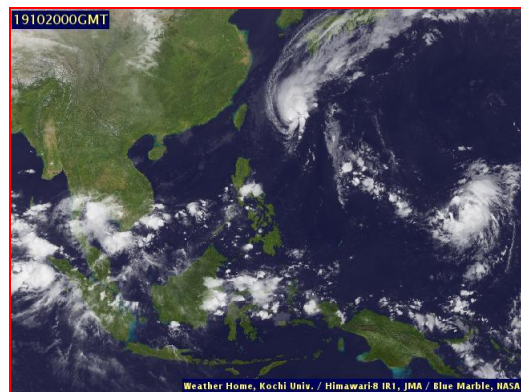
ภาพถ่ายจากดาวเทียม วันที่ 20 ต.ค. 2562
