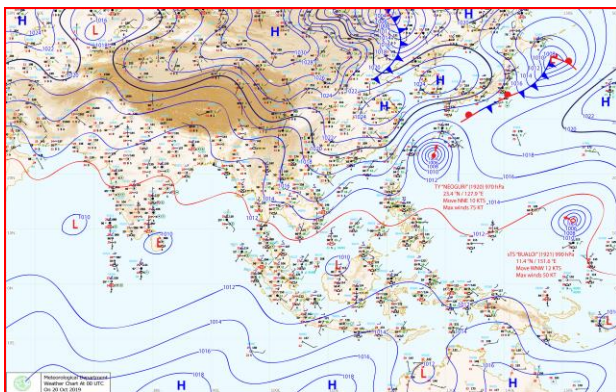
แผนที่อากาศ วันที่ 20 ต.ค. 2562 เวลา 07.00 น.
