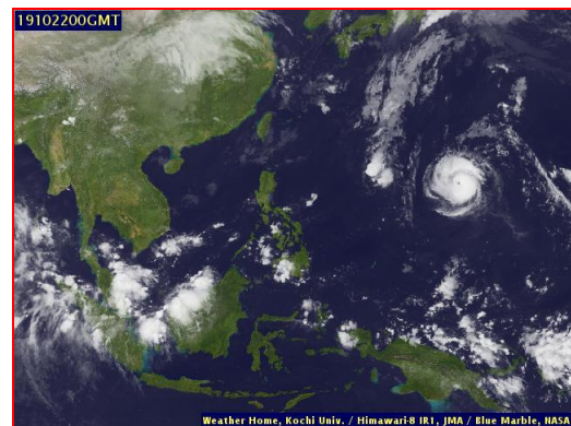
ภาพถ่ายจากดาวเทียม วันที่ 22 ต.ค. 2562
