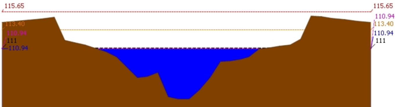
▲ ระดับปัจจุบัน --- ระดับวิกฤติ --- ระดับฝายระวัง ---- เมื่อกาน 7:00 น. - - - - คาคการลลวงหน้า 1 วัน สถานี 120107T แม่น้ำป่าสักที่ อ.เมืองเพชรบูรณ์ ต.นาป่า อ.เมือง จ.เพชรบูรณ์ ระดับน้ำ 110.94 ม.รทก.
