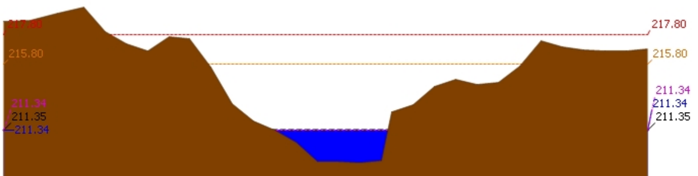
▲ ระดับปัจจุบัน --- ระดับวิกฤติ --- ระดับฝายระวัง ---- เมื่อกาน 7:00 น. - - - - คาคการลลวงหน้า 1 วัน สถานี 120205T แม่น้ำป่าสักที่ บ้านลุ่มกะทาด ต.ศิลา อ.หล่มเก่า จ.เพชรบูรณ์ ระดับน้ำ 211.34 ม.รทก.
