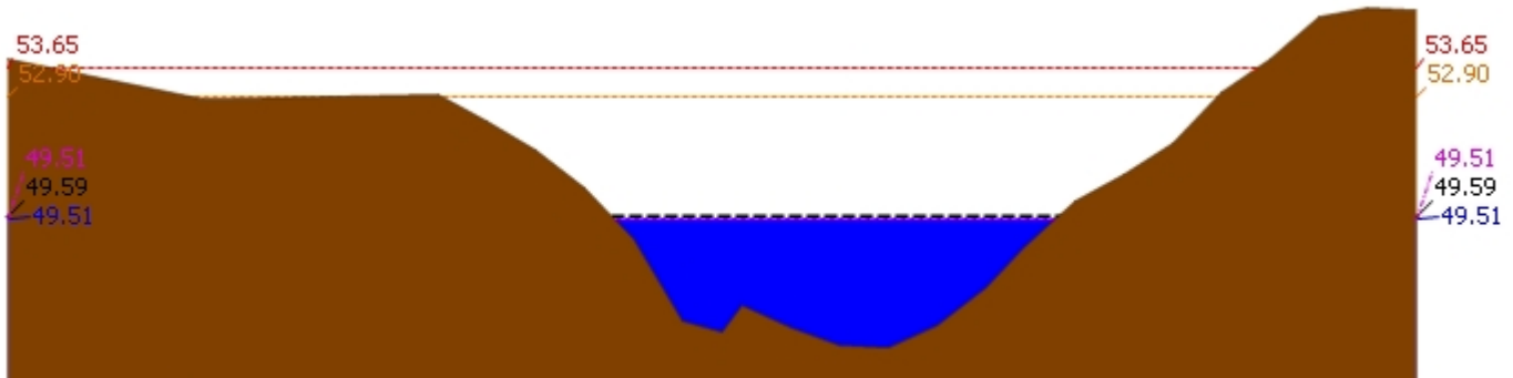
▲ ระดับปัจจุบัน --- ระดับวิกฤติ --- ระดับฝายระวัง ---- เมื่อวาน 7:00 น. - - - - - คาดการณ์ล่วงหน้า 1 วัน สถานี 120113T แม่น้ำป่าสักที่บ้านเขาค้าง ต.คลองกระจิง อ.ศรีเทพ จ.เพชรบูรณ์ ระดับน้ำ 49.51 ม.รทก.
