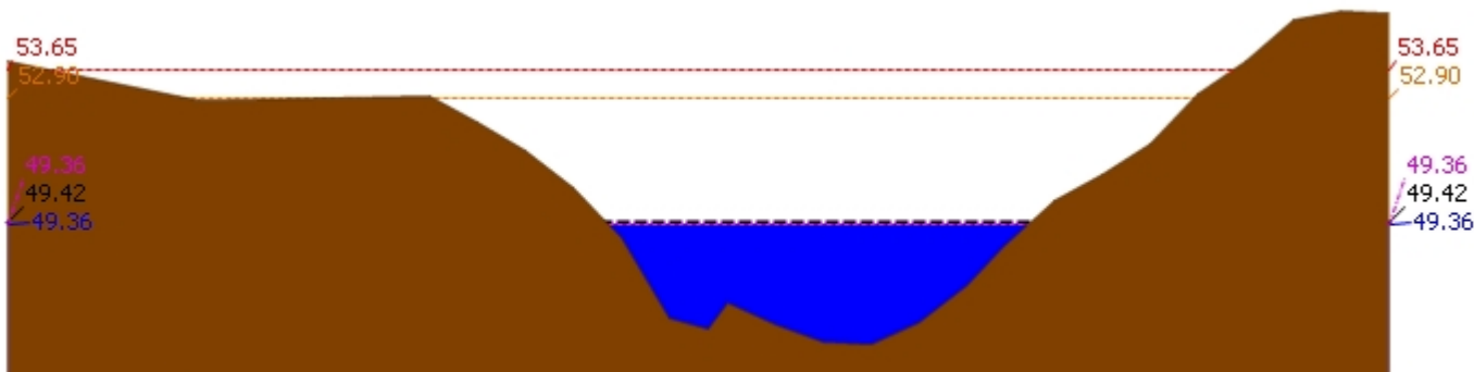
▲ ระดับปัจจุบัน --- ระดับวิกฤติ --- ระดับเฝ้าระวัง ---- เมื่อกวาน 7:00 น. - - - - คาดการณ์ล่วงหน้า 1 วัน สถานี 120113T แม่น้ำป่าสักที่บ้านเขาค้าง ต.คลองกระจิง อ.ศรีเทพ จ.เพชรบูรณ์ ระดับน้ำ 49.36 ม.รทก.
