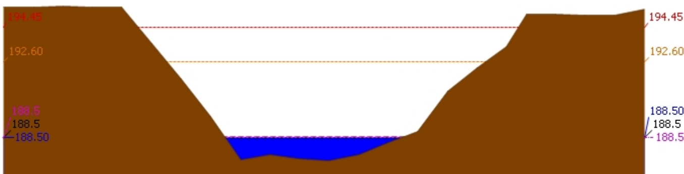
▲ ระดับปัจจุบัน --- ระดับวิกฤติ --- ระดับเฝ้าระวัง ---- เมื่อกวาน 7:00 น. - - - - คาดการณ์ล่วงหน้า 1 วัน สถานี 120901T ห้วยมวกเหล็กที่ อ.มวกเหล็ก ต.มวกเหล็ก อ.มวกเหล็ก จ.สระบุรี ระดับน้ำ 188.50 ม.รทก.
