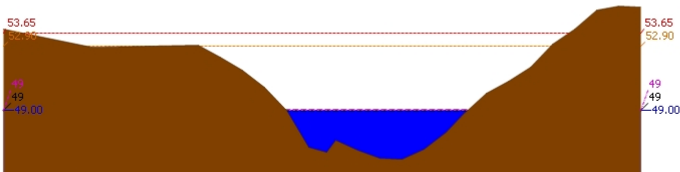
▲ ระดับปัจจุบัน --- ระดับวิกฤติ --- ระดับฝายระวัง ---- เมื่อกวาน 7:00 น. - - - - คาคการลลวงหน้า 1 วัน สถานี 120113T แม่น้ำป่าสักที่บ้านเขาค้าง ต.คลองกระจิง อ.ศรีเทพ จ.เพชรบูรณ์ ระดับน้ำ 49.00 ม.รทก.
