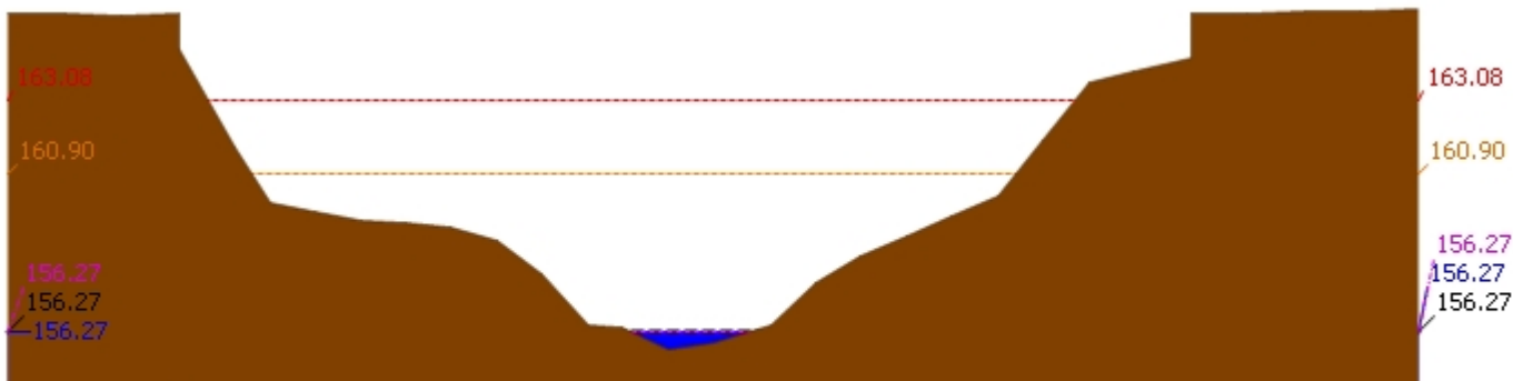
▲ ระดับปัจจุบัน --- ระดับวิกฤติ --- ระดับเฝ้าระวัง ---- เมื่อกว่า 7:00 น. - - - - - คาดการณ์ล่วงหน้า 1 วัน สถานี 120105T แม่น้ำป่าสักที่บ้านวังมเสหนือ ต.ท่าอิฐ อ.หล่มสัก จ.เพชรบูรณ์ ระดับน้ำ 156.27 ม.รทก.
