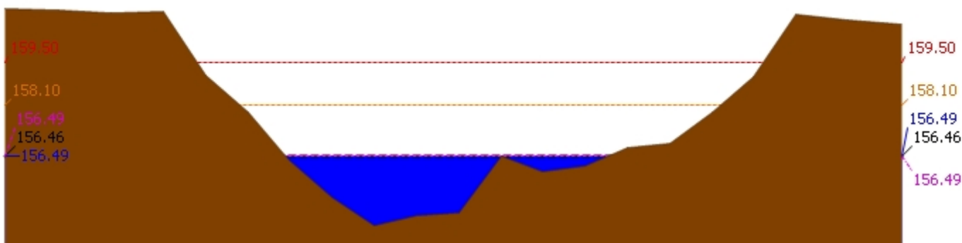
▲ ระดับปัจจุบัน --- ระดับวิกฤติ --- ระดับเฝ้าระวัง ---- เมื่อกว่า 7:00 น. - - - - - คาดการณ์ล่วงหน้า 1 วัน สถานี 120305T หัวน้ำพุที่ อ.หล่มเก่า ต.หล่มเก่า อ.หล่มเก่า จ.เพชรบูรณ์ ระดับน้ำ 156.49 ม.รทก.
