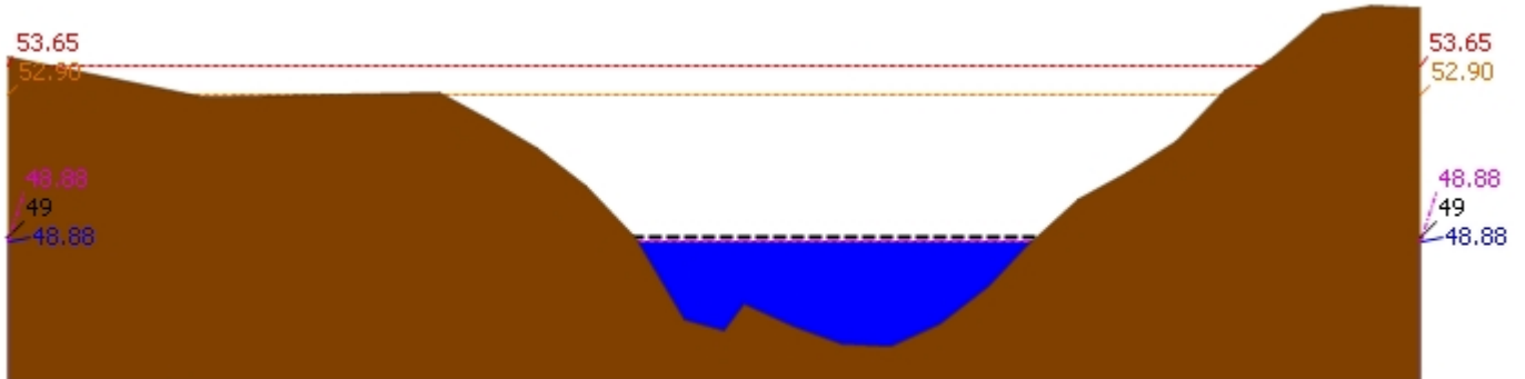
▲ ระดับปัจจุบัน --- ระดับวิกฤติ --- ระดับเฝ้าระวัง ---- เมื่อกวาน 7:00 น. - - - - คาดการณ์ล่วงหน้า 1 วัน สถานี 120113T แม่น้ำป่าสักที่บ้านเขาค้าง ต.คลองกระจิง อ.ศรีเทพ จ.เพชรบูรณ์ ระดับน้ำ 48.88 ม.รทก.
