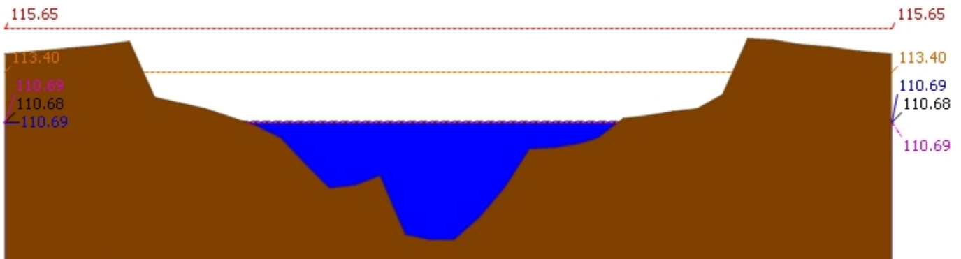
▲ ระดับปัจจุบัน --- ระดับวิกฤติ --- ระดับเฟิาระวัง ---- เมื่อกาน 7:00 น. - - - - คาคการล้ลวงหน้า 1 วัน สถานี 120107T แม่น้ำป่าสักที่ อ.เมืองเพชรบูรณ์ ต.นาป่า อ.เมือง จ.เพชรบูรณ์ ระดับน้ำ 110.69 ม.รทก.
