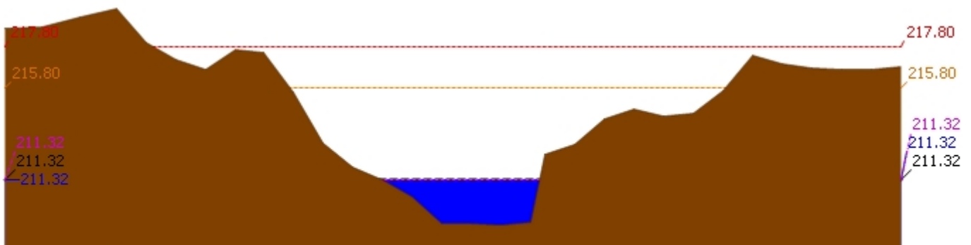
▲ ระดับปัจจุบัน --- ระดับวิกฤติ --- ระดับเฟิาระวัง ---- เมื่อกาน 7:00 น. - - - - คาคการล้ลวงหน้า 1 วัน สถานี 120205T แม่น้ำป่าสักที่ บ้านอุมกะทาด ต.ศิลา อ.หล่มเก่า จ.เพชรบูรณ์ ระดับน้ำ 211.32 ม.รทก.
