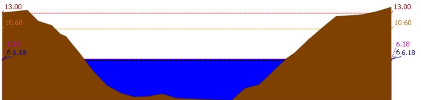
▲ ระดับปัจจุบัน --- ระดับวิกฤติ --- ระดับเฟิาระวัง ---- เมื่อกาน 7:00 น. - - - - คาคการล้ลวงหน้า 1 วัน สถานี 120106T แม่น้ำป่าสักที่ อ.เสาให้ ต.ศาลาริไทย อ.เสาให้ จ.สระบุรี ระดับน้ำ 6.18 ม.รทก.
