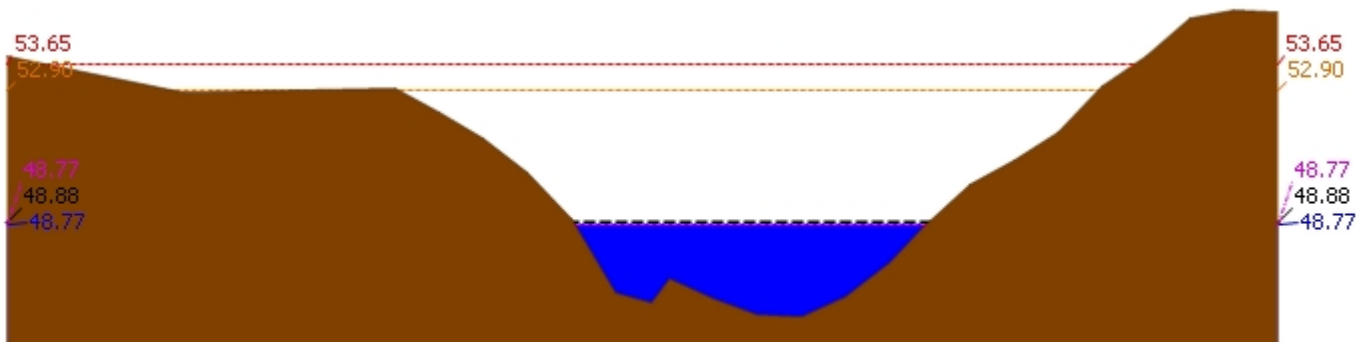
▲ ระดับปัจจุบัน --- ระดับวิกฤติ --- ระดับฝายระวัง ---- เมื่อวาน 7:00 น. - - - - คาดการณ์ล่วงหน้า 1 วัน สถานี 120113T แม่น้ำป่าสักที่บ้านเขาค้าง ต.คลองกระจิง อ.ศรีเทพ จ.เพชรบูรณ์ ระดับน้ำ 48.77 ม.รทก.
