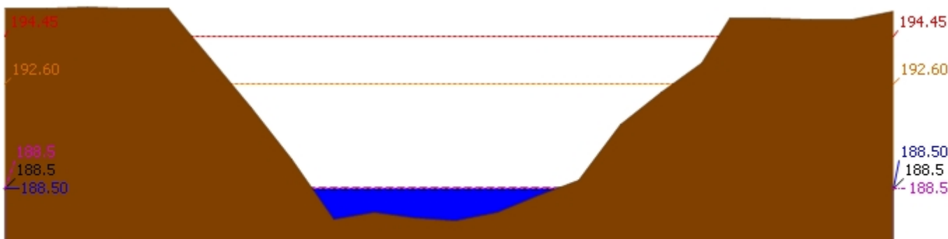
▲ ระดับปัจจุบัน --- ระดับวิกฤติ --- ระดับฝายระวัง ---- เมื่อวาน 7:00 น. - - - - คาดการณ์ล่วงหน้า 1 วัน สถานี 120901T ห้วยมวกเหล็กที่ อ.มวกเหล็ก ต.มวกเหล็ก อ.มวกเหล็ก จ.สระบุรี ระดับน้ำ 188.50 ม.รทก.
