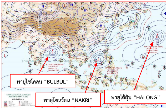
แผนที่อากาศ วันที่ ๘ พ.ย. ๒๕๖๒ เวลา ๐๗.๐๐ น.
