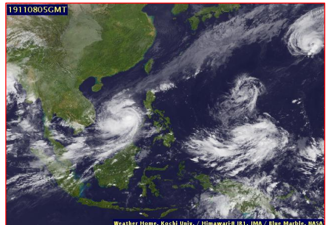
ภาพถ่ายดาวเทียม วันที่ ๘ พ.ย. ๒๕๖๒ เวลา ๑๒.๐๐ น.
