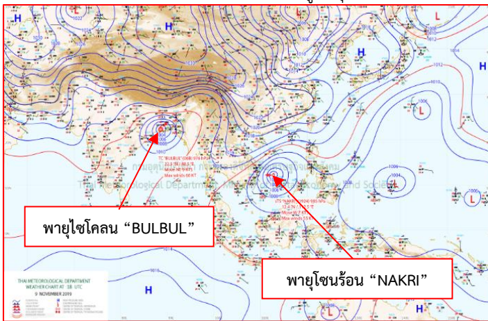
แผนที่อากาศ วันที่ ๑๐ พ.ย. ๒๕๖๒ เวลา ๐๑.๐๐ น.
