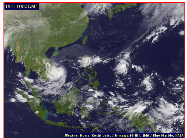
ภาพถ่ายดาวเทียม วันที่ ๑๐ พ.ย. ๒๕๖๒ เวลา ๐๗.๐๐ น.
