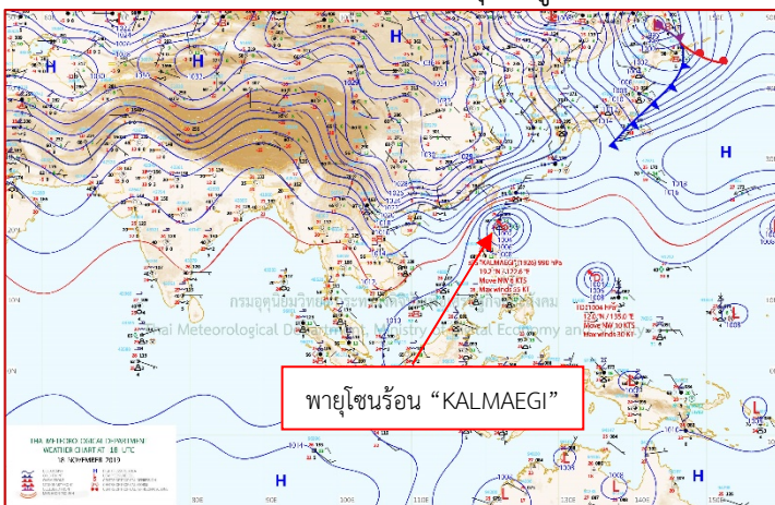
แผนที่อากาศ วันที่ ๑๙ พ.ย. ๒๕๖๒ เวลา ๐๑.๐๐ น.
