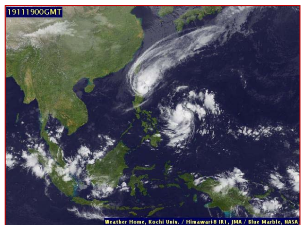
ภาพถ่ายดาวเทียม วันที่ ๑๙ พ.ย. ๒๕๖๒ เวลา ๐๗.๐๐ น.
