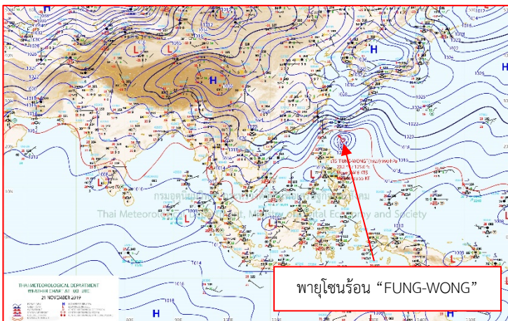
แผนที่อากาศ วันที่ ๒๑ พ.ย. ๒๕๖๒ เวลา ๐๗.๐๐ น.
