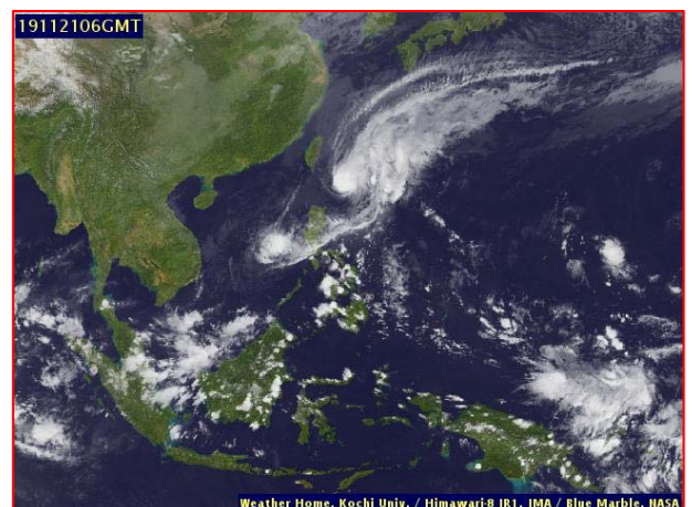
ภาพถ่ายดาวเทียม วันที่ ๒๑ พ.ย. ๒๕๖๒ เวลา ๑๓.๐๐ น.
