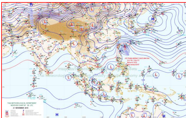
แผนที่อากาศ วันที่ 22 พ.ย. 2562 เวลา 01.00 น.
