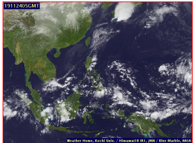
ภาพถ่ายดาวเทียม วันที่ ๒๔ พ.ย. ๒๕๖๒ เวลา ๑๓.๐๐ น.
