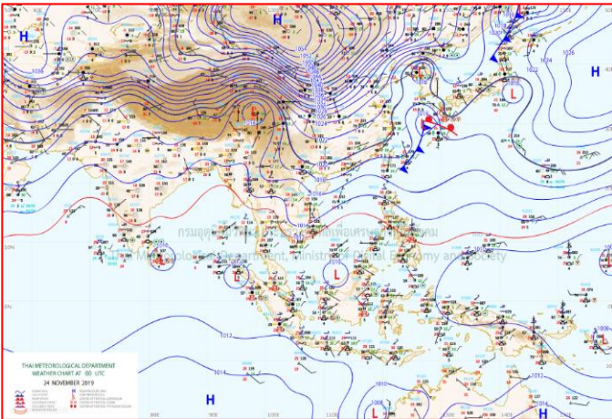
แผนที่อากาศ วันที่ ๒๔ พ.ย. ๒๕๖๒ เวลา ๐๗.๐๐ น.
