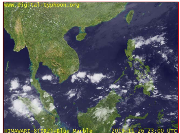
ภาพถ่ายดาวเทียม วันที่ ๒๗ พ.ย. ๒๕๖๒ เวลา ๐๖.๐๐ น.
