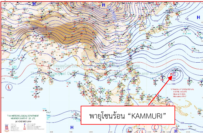
แผนที่อากาศ วันที่ ๒๗ พ.ย. ๒๕๖๒ เวลา ๐๑.๐๐ น.
