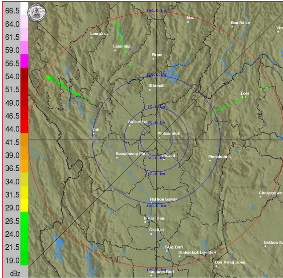
ภาพเรดาร์ตรวจอากาศ “พิษณุโลก” ณ วันที่ 28 พฤศจิกายน 2562 (ที่มา : กรมอุตุนิยมวิทยา)
