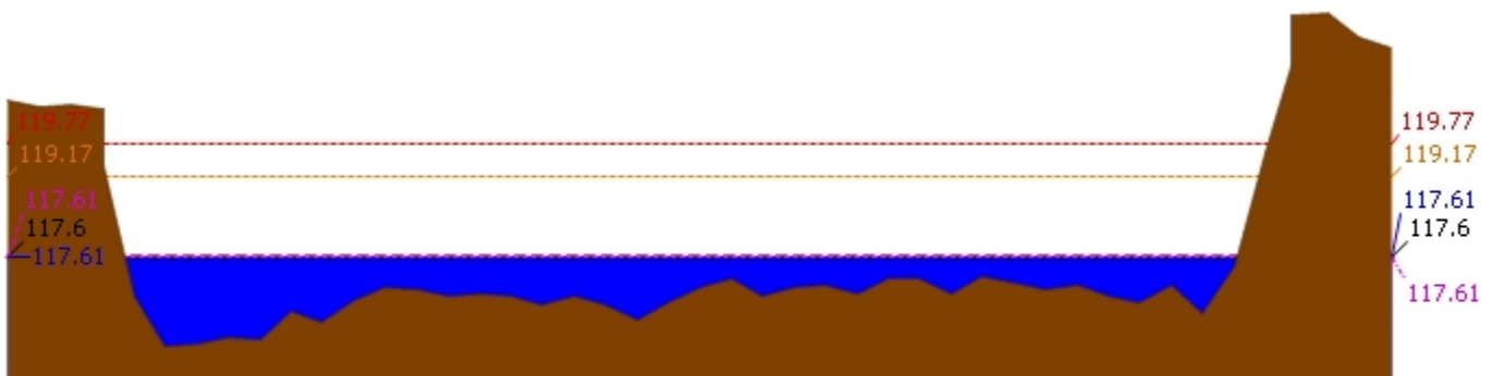
▲ ระดับปัจจุบัน --- ระดับวิกฤติ --- ระดับฝายระวัง ---- เมื่อวาน 7:00 น. - - - - - คาดการณ์ล่วงหน้า 1 วัน สถานี 060111T แม่น้ำปิงที่บ้านปากร่องห้วยจี่ ต.ตากออก อ.บ้านตาก จ.ตาก ระดับน้ำ 117.61 ม.รทก.
