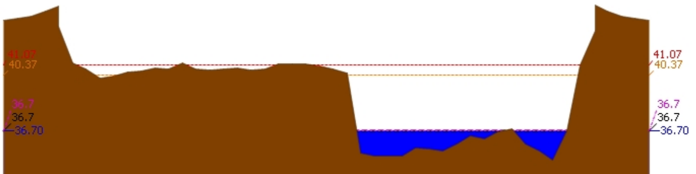
▲ ระดับปัจจุบัน --- ระดับวิกฤติ --- ระดับฝายระวัง ---- เมื่อวาน 7:00 น. - - - - - คาดการณ์ล่วงหน้า 1 วัน สถานี 060110T แม่น้ำปิงที่บ้านบางแก้ว ต.บางแก้ว อ.บรรพตพิสัย จ.นครสวรรค์ ระดับน้ำ 36.70 ม.รทก.
