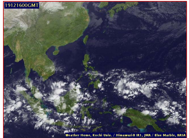
ภาพถ่ายดาวเทียม วันที่ ๑๖ ธ.ค. ๒๕๖๒ เวลา ๐๗.๐๐ น.
