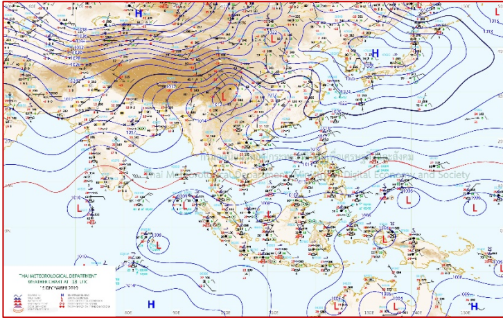
แผนที่อากาศ วันที่ ๑๖ ธ.ค. ๒๕๖๒ เวลา ๐๖.๐๐ น.
