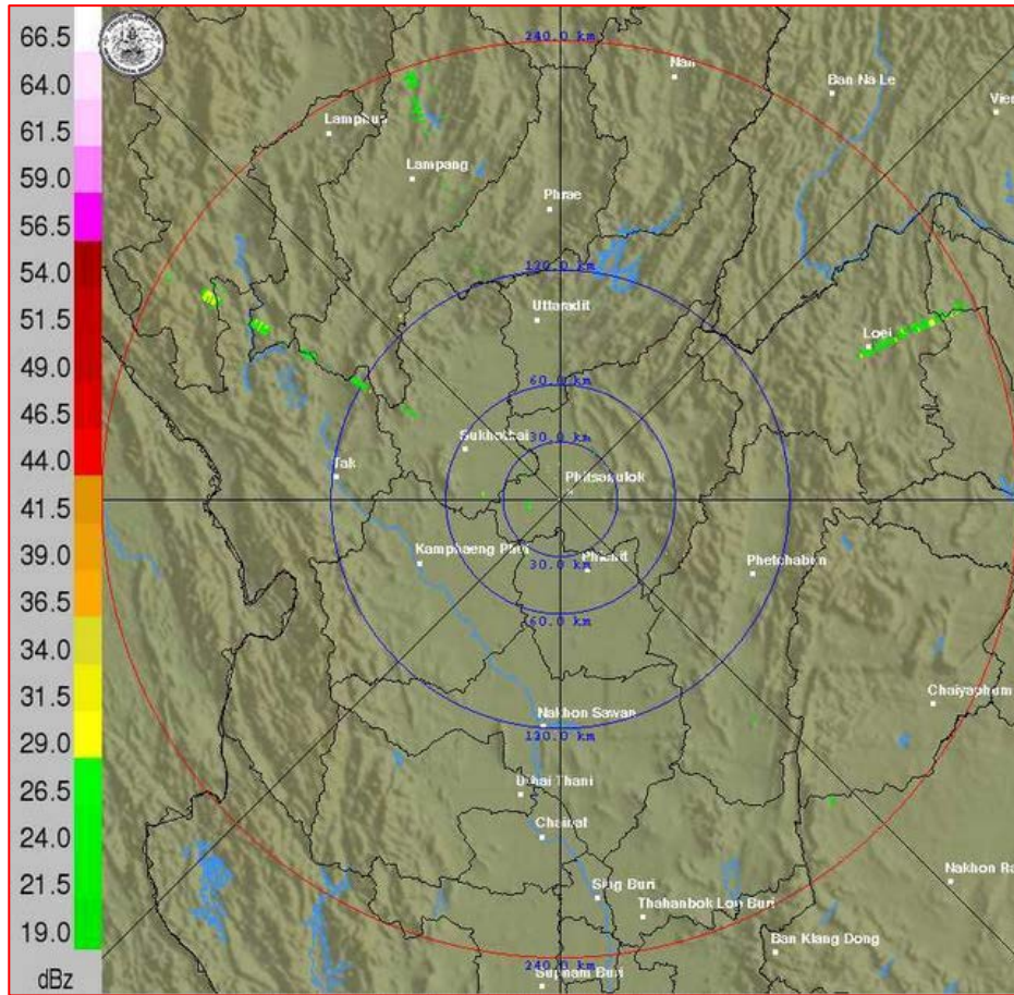
ภาพเรดาร์ตรวจอากาศ “พิชญ์โลก” ณ วันที่ 6 มกราคม 2563 (ที่มา : กรมอุตุนิยมวิทยา)
