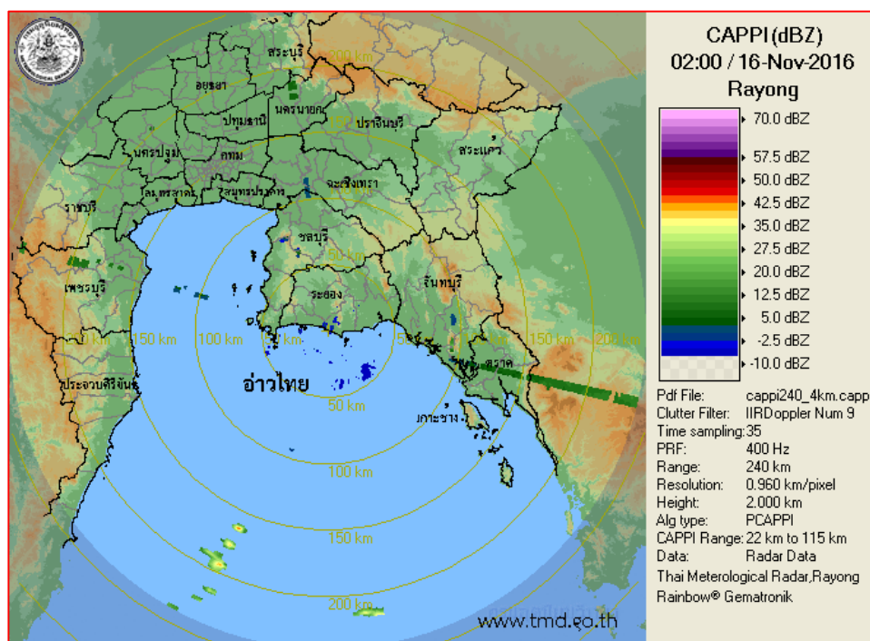
ภาพเรดาร์ตรวจอากาศ “ระยอง” ณ วันที่ 16 พฤศจิกายน 2559 (ที่มา : กรมอุตุนิยมวิทยา)
