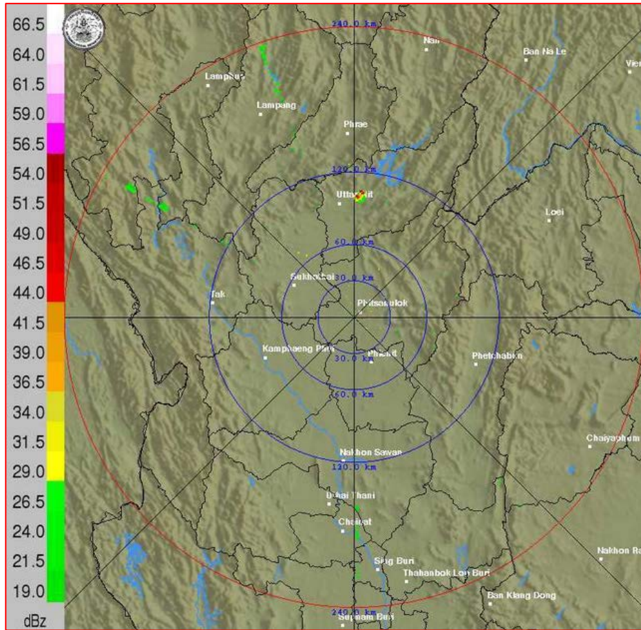
ภาพเรดาร์ตรวจอากาศ “พิชญ์โลก” ณ วันที่ 14 มกราคม 2563 (ที่มา : กรมอุตุนิยมวิทยา)
