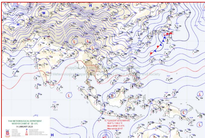
แผนที่อากาศ วันที่ ๑๕ ม.ค. ๒๕๖๓ เวลา ๐๖.๐๐ น.
