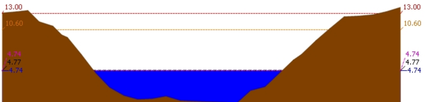
▲ ระดับปัจจุบัน --- ระดับวิกฤติ --- ระดับเฝ้าระวัง ---- เมื่อวาน 7:00 น. - - - - - คาดการณ์ล่วงหน้า 1 วัน สถานี 120106T แม่น้ำป่าสักที่ อ.เสนาห์ ต.ศาลาวิไทย อ.เสนาห์ จ.สระบุรี ระดับน้ำ 4.74 ม.รทก.
