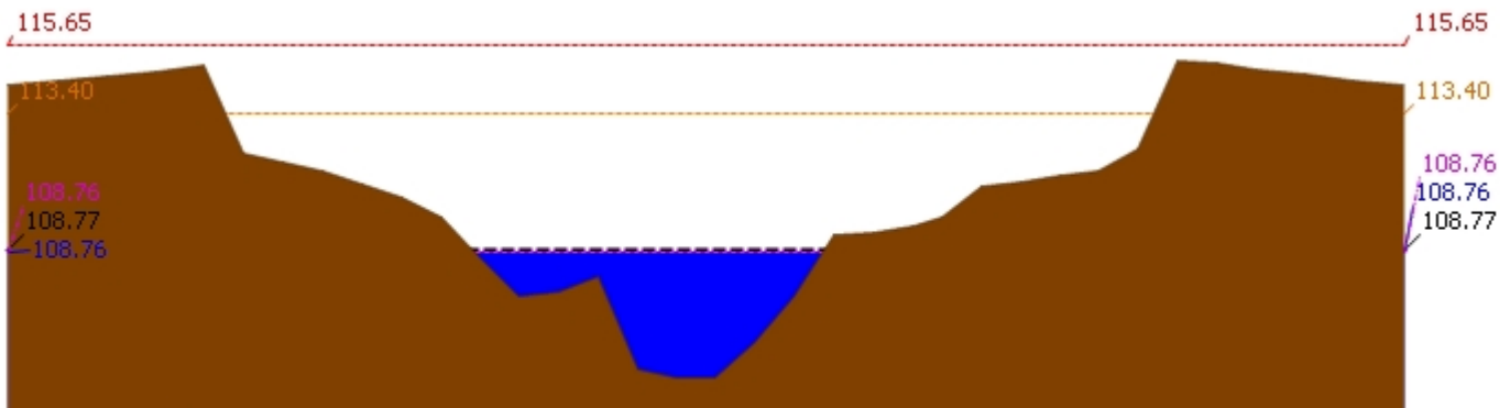
▲ ระดับปัจจุบัน --- ระดับวิกฤติ --- ระดับเฝ้าระวัง ---- เมื่อวาน 7:00 น. - - - - - คาดการณ์ล่วงหน้า 1 วัน สถานี 120107T แม่น้ำป่าสักที่ อ.เมืองเพชรบูรณ์ ต.นาป่า อ.เมือง จ.เพชรบูรณ์ ระดับน้ำ 108.76 ม.รทก.
