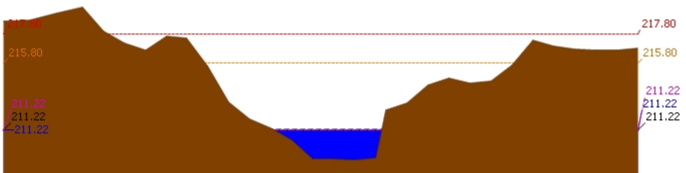
▲ ระดับปัจจุบัน --- ระดับวิกฤติ --- ระดับเฝ้าระวัง ---- เมื่อวาน 7:00 น. - - - - - คาดการณ์ล่วงหน้า 1 วัน สถานี 120205T แม่น้ำป่าสักที่บ้านอุมกะทาด ต.ศิลา อ.หล่มเก่า จ.เพชรบูรณ์ ระดับน้ำ 211.22 ม.รทก.
