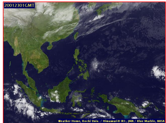
ภาพถ่ายจากดาวเทียม วันที่ 23 ม.ค. 2563
