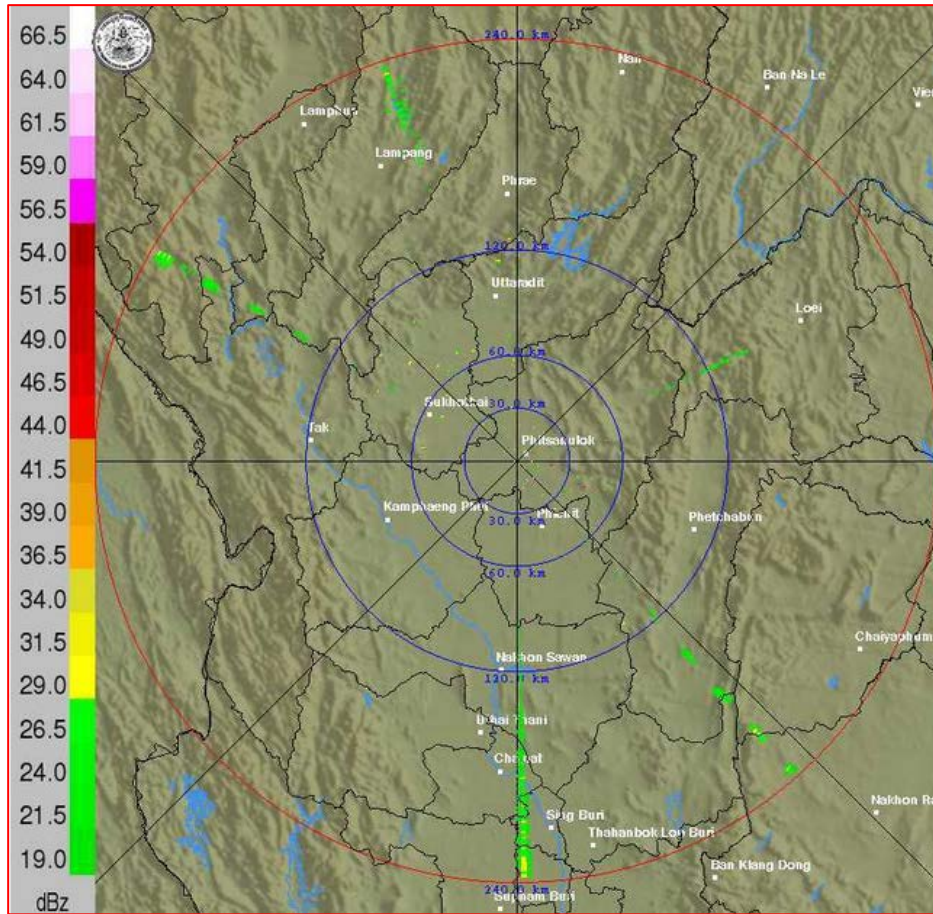
ภาพเรดาร์ตรวจอากาศ “พิชญ์โลก” ณ วันที่ 23 มกราคม 2563 (ที่มา : กรมอุตุนิยมวิทยา)
