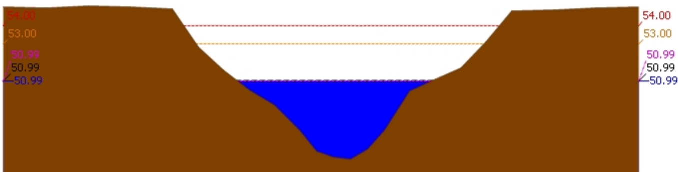
▲ ระดับปัจจุบัน --- ระดับวิกฤติ --- ระดับ الفيضان ---- เมื่อกวาน 7:00 น. - - - - คาดการณ์ล่วงหน้า 1 วัน สถานี 120702T ลำสนธิที่บ้านท่าช้าง ต.หนองขาหย่าง อ.ชัยบาดาล จ.ลพบุรี ระดับน้ำ 50.99 ม.รทก.
