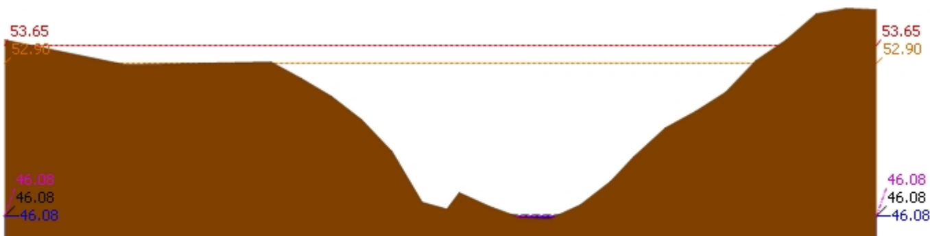
▲ ระดับปัจจุบัน --- ระดับวิกฤติ --- ระดับ الفيضان ---- เมื่อกวาน 7:00 น. - - - - คาดการณ์ล่วงหน้า 1 วัน สถานี 120113T แม่น้ำป่าสักที่บ้านเขาค้าง ต.คลองกระจิง อ.ศรีเทพ จ.เพชรบูรณ์ ระดับน้ำ 46.08 ม.รทก.
